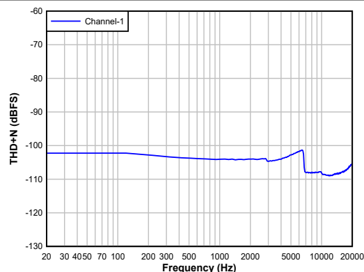
差分接收器输出, 32 \Omega 负载 ( -1dBFS 输入 )
