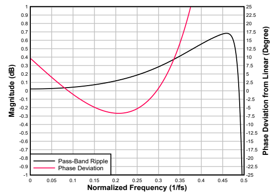
图 6-51. 超低延迟抽取滤波器通带纹波和相位偏差
