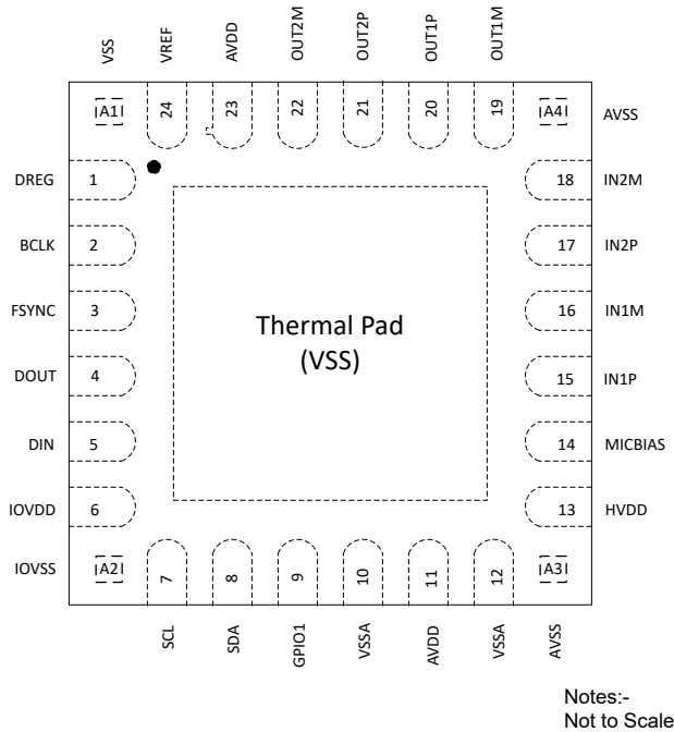
图 4-1. TAC5301-Q1 带有外露散热焊盘和转角引脚的 24 引脚 QFN 封装，顶视图
