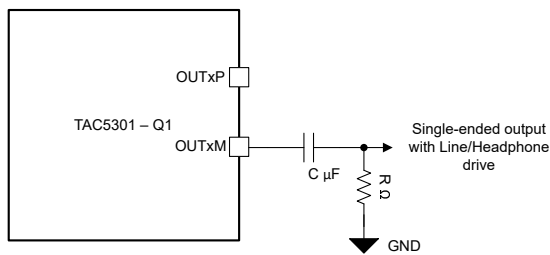
图 6-21. OUT1M 上的单声道单端输出连接 (OUT1x_CFG[2:0] = 3'b011)
