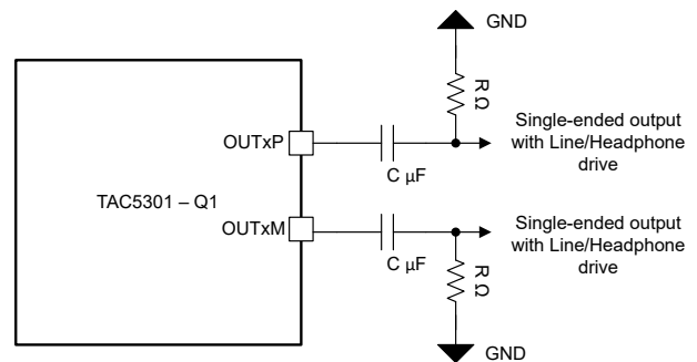
图 6-22. 立体声单端输出连接 (OUT1x_CFG[2:0] = 3'b001)
