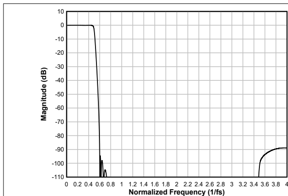
图 6-81. 低延迟内插滤波器幅度响应
