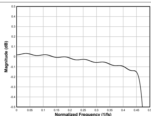
图 6-64. 线性相位内插滤波器通带纹波
