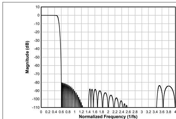
图 6-63. 线性相位内插滤波器幅度响应
