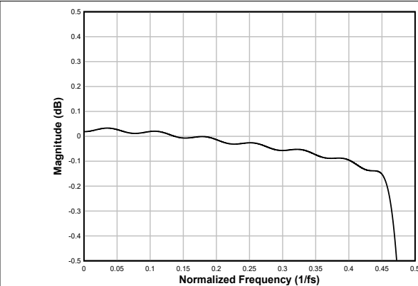
图 6-66. 线性相位内插滤波器通带纹波
