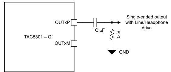
图 6-20. OUT1P 上的单声道单端输出连接 (OUT1x_CFG[2:0] = 3'b010)
