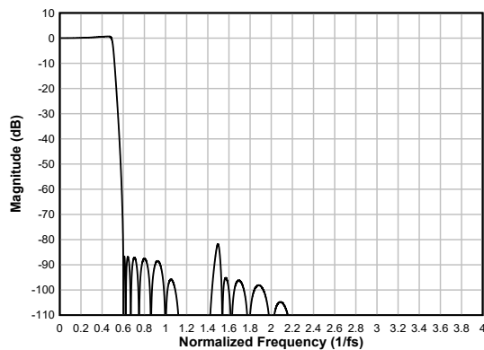
图 6-50. 超低延迟抽取滤波器幅度响应
