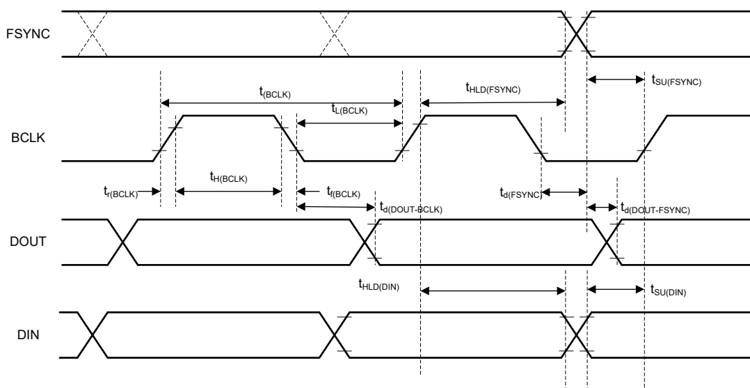
图 5-2. TDM (其中 BCLK_POL = 1)、I 2 S 和 LJ 接口时序图
