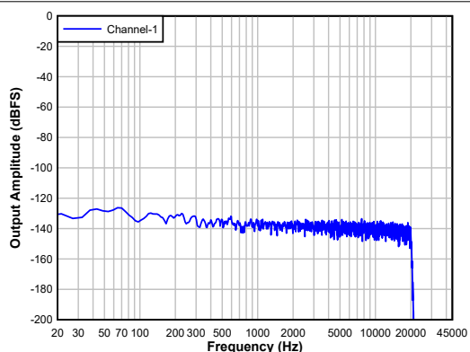
差分输出
