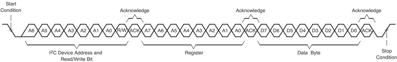
图 6-98. I 2 C 单字节写入传输
