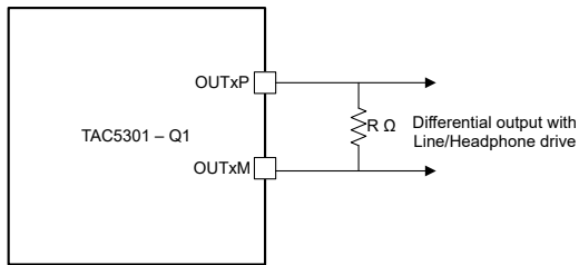
图 6-19. 差分输出连接 (OUT1x_CFG[2:0] = 3'b000)
