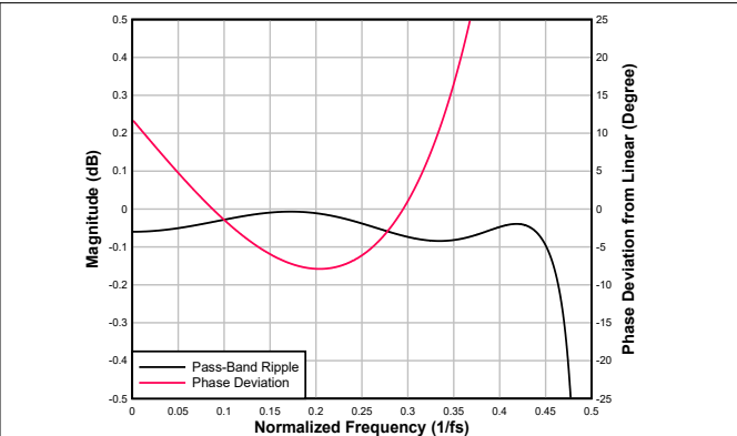
图 6-90. 超低延迟内插滤波器通带纹波和相位偏差
