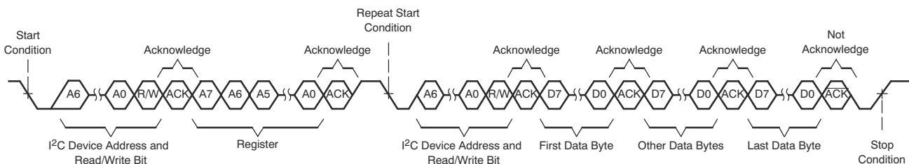
图 6-101. I 2 C 多字节读取传输
