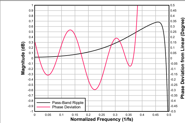
图 6-41. 低延迟抽取滤波器通带纹波和相位偏差
