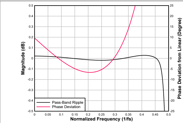
图 6-57. 超低延迟抽取滤波器通带纹波和相位偏差
