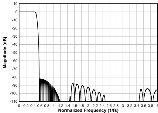
图 7-36. 线性相位内插滤波器幅度响应
