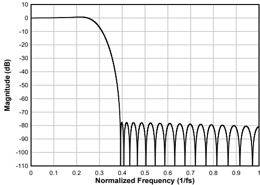
图 7-44. 线性相位内插滤波器幅度响应
