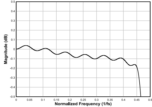
图 7-43. 线性相位内插滤波器通带纹波
