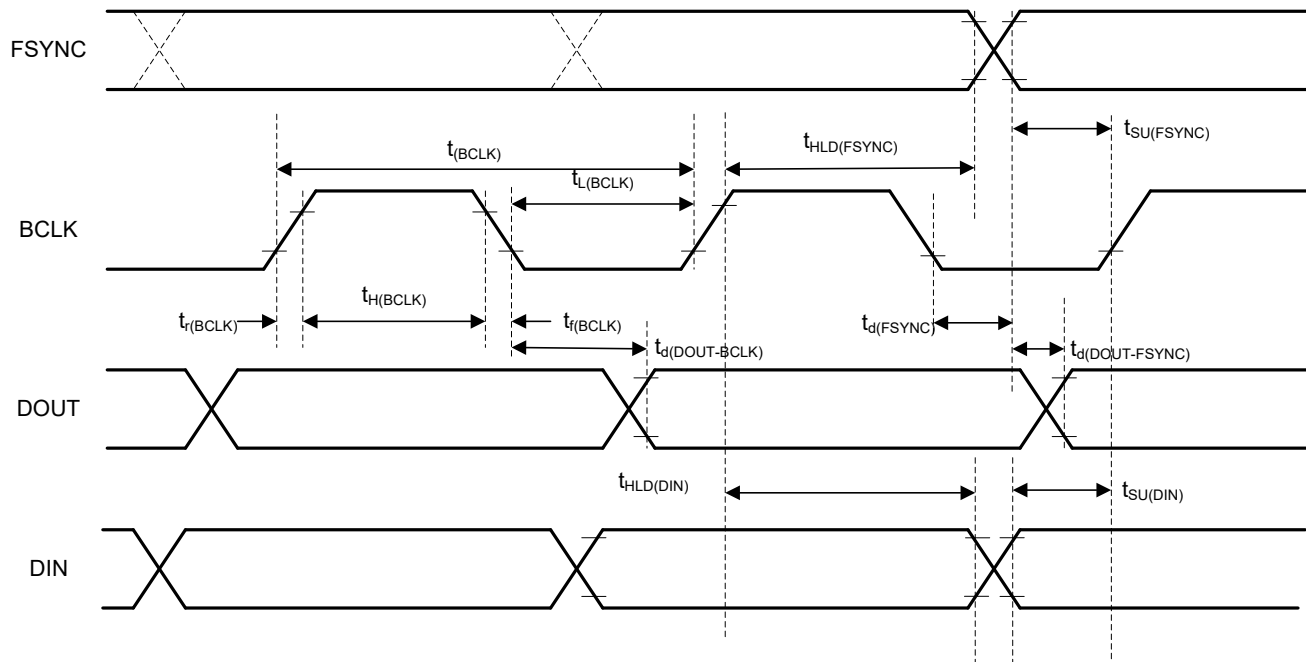
图 6-3. TDM (其中 BCLK_POL = 1)、I²S 和 LJ 接口时序图
