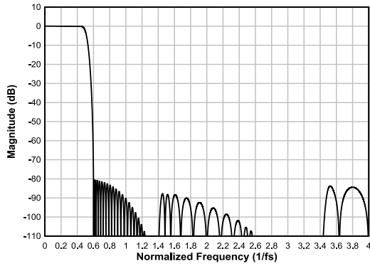
图 7-34. 线性相位内插滤波器幅度响应
