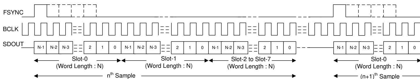
图 7-5. TDM 模式协议时序 (PASI_TX_OFFSET = 0 且 PASI_BCLK_POL = 1)
