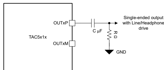
图 7-22. OUT1P 上的单声道单端输出连接 (OUT1x_CFG[2:0] = 3'b010)
