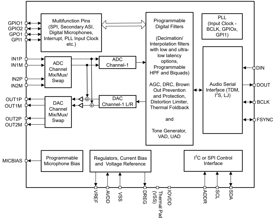
图 7-1. 功能方框图
