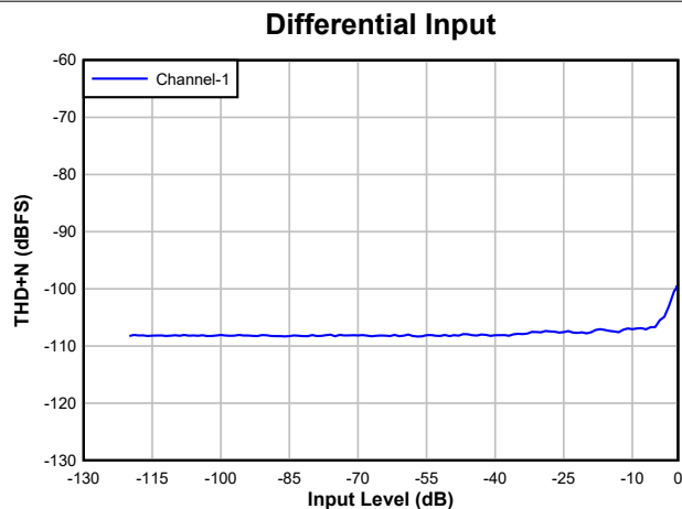
图 6-6. ADC THD+N 级别与输入间的关系
