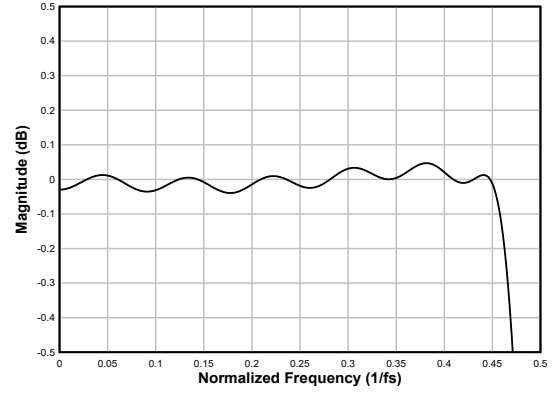
图 7-37. 线性相位抽取滤波器通带纹波
