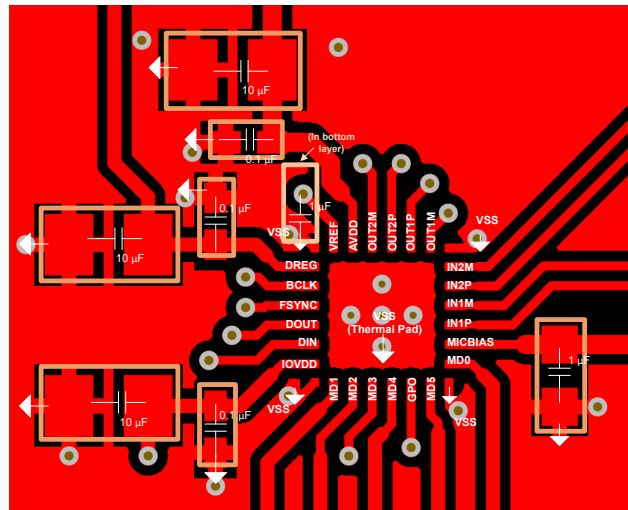
图 8-7. 示例布局
