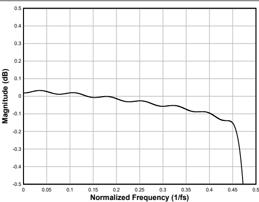
图 6-74. 线性相位内插滤波器通带纹波
