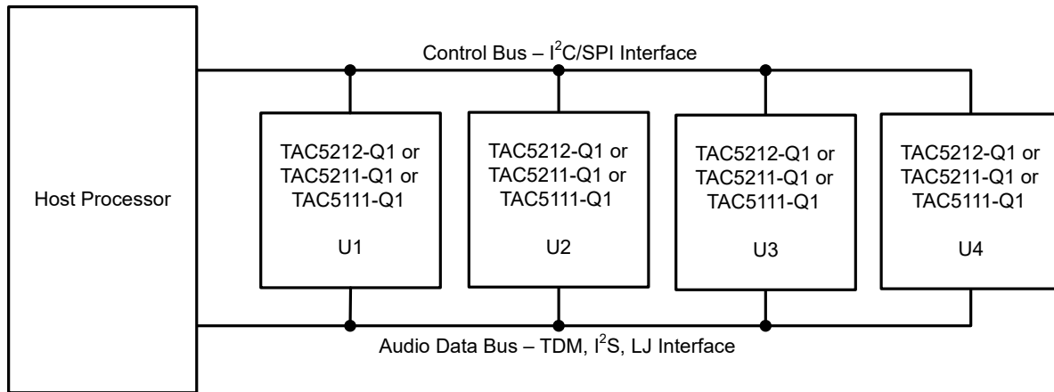
图 6-14. 多个 TAC5112-Q1 器件具有共享控制和音频数据总线
