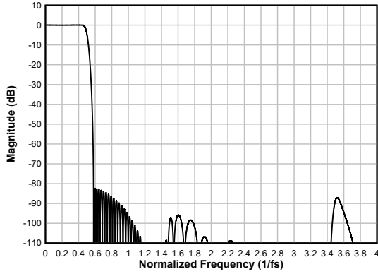
图 6-40. 线性相位抽取滤波器幅度响应
