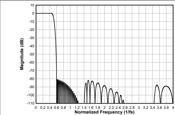
图 6-36. 线性相位抽取滤波器幅度响应
