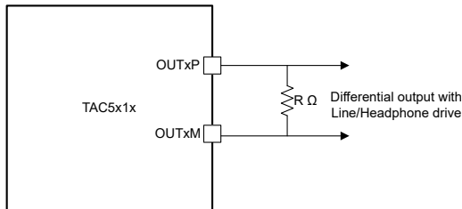
图 6-21. 差分输出连接 (OUT1x_CFG[2:0] = 3'b000)
