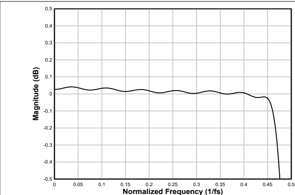
图 6-31. 线性相位抽取滤波器通带纹波
