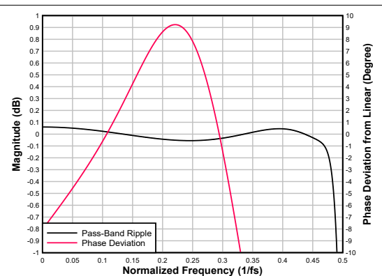
图 6-57. 低延迟抽取滤波器通带纹波和相位偏差
