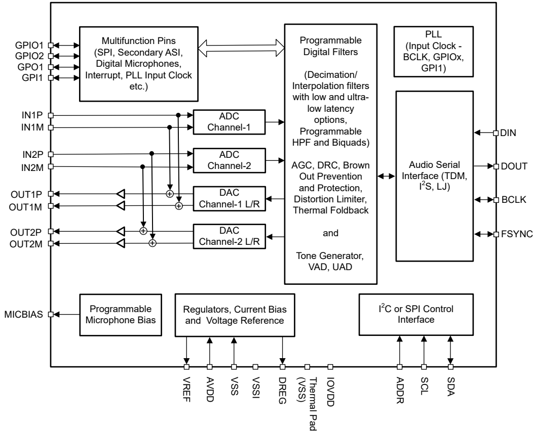
图 6-1. 功能方框图
