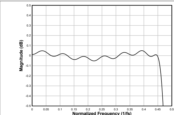
图 6-39. 线性相位抽取滤波器通带纹波
