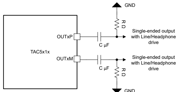
图 6-24. 立体声单端输出连接 (OUT1x_CFG[2:0] = 3'b001)
