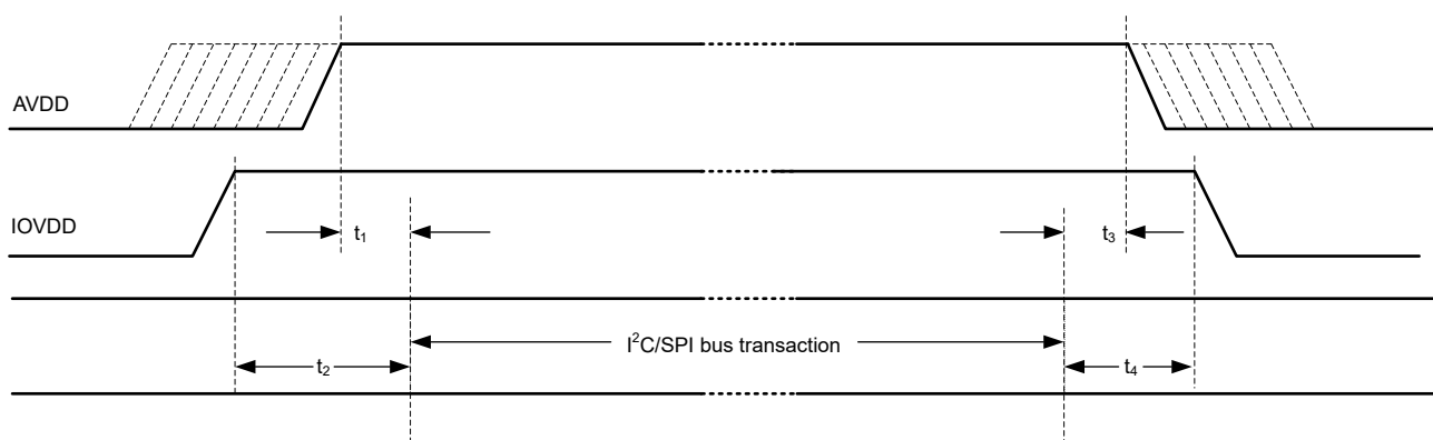
图 8-6. 电源时序要求时序图
