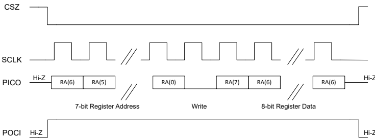
图 6-114. SPI 单字节写入传输
