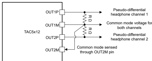
图 6-23. 带外部共模检测的伪差分输出连接 (OUT1x_CFG[2:0] = 3'b101)
