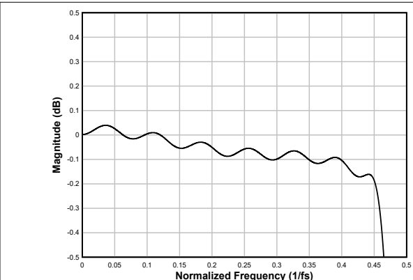
图 6-82. 线性相位内插滤波器通带纹波
