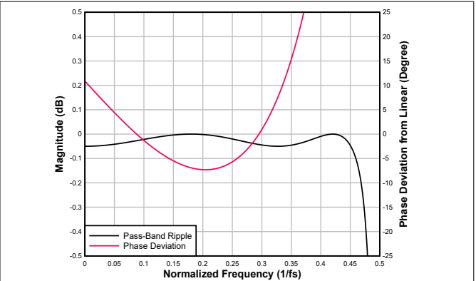
图 6-106. 超低延迟内插滤波器通带纹波和相位偏差
