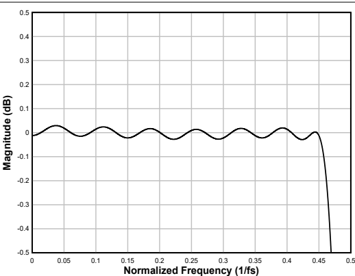
图 6-76. 线性相位内插滤波器通带纹波
