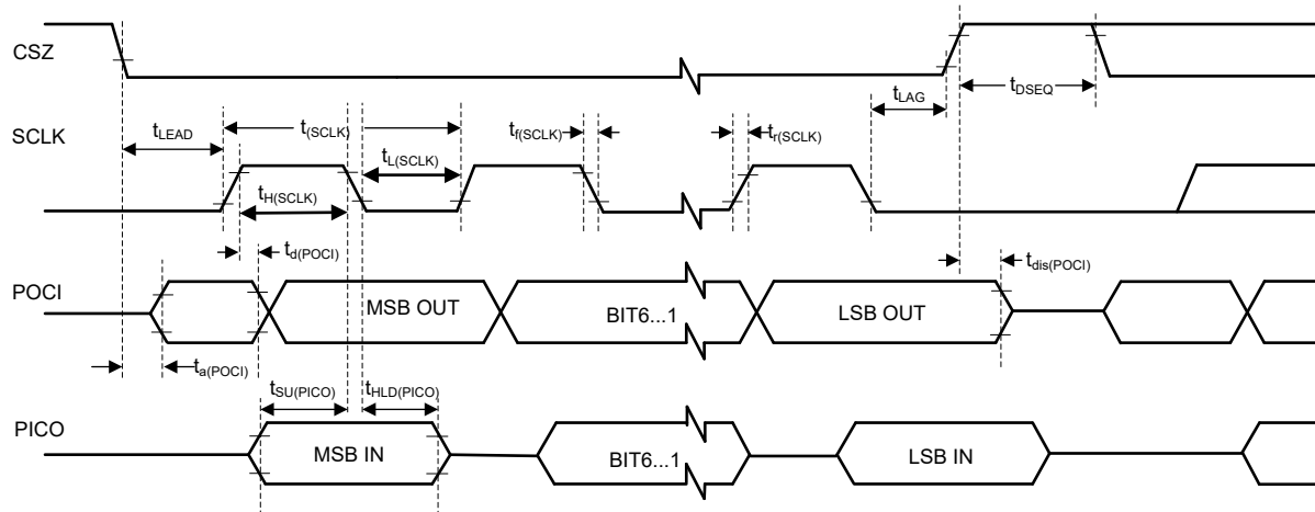
图 5-2. SPI 时序图
