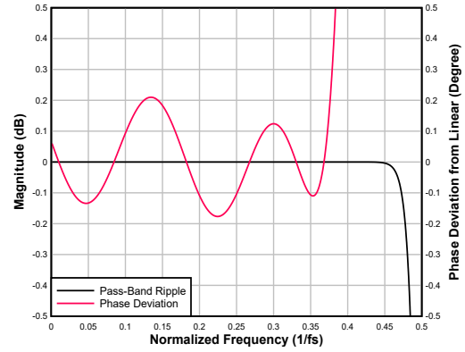
图 6-98. 低延迟内插滤波器通带纹波和相位偏差
