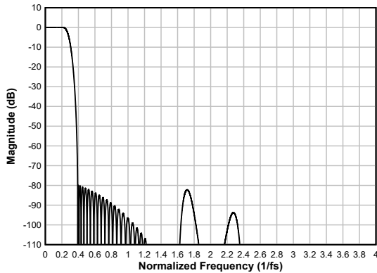
图 6-42. 线性相位抽取滤波器幅度响应
