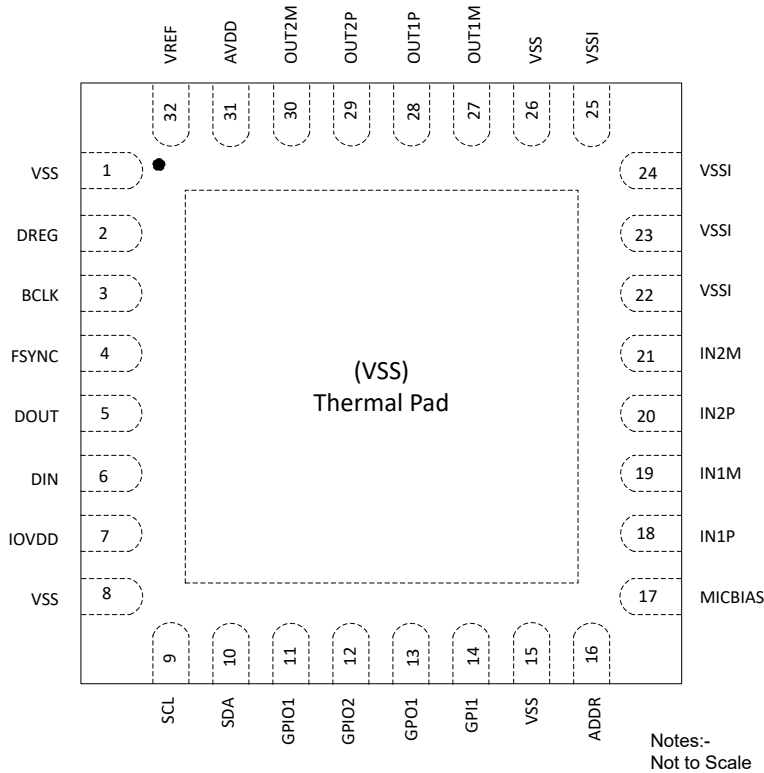
图 4-1. TAC5112-Q1 RTV 封装，32 引脚 WQFN ( 带有外露散热焊盘 )，顶视图
