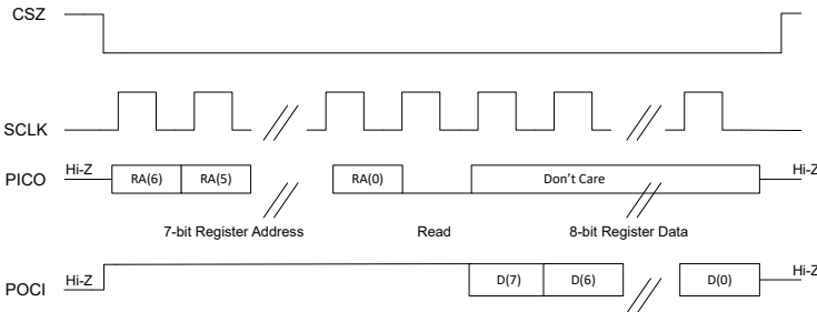
图 6-115. SPI 单字节读取传输
