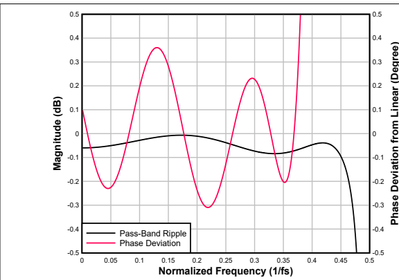
图 6-94. 低延迟内插滤波器通带纹波和相位偏差
