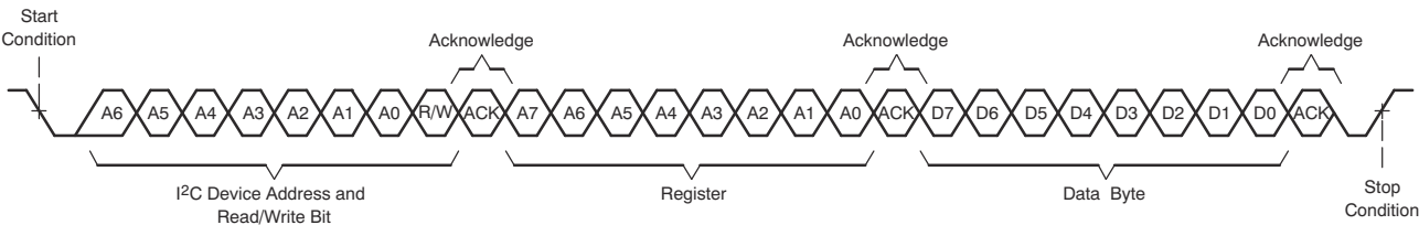
图 6-110. I²C 单字节写入传输
