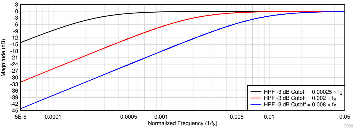
图 6-70. HPF 滤波器频率响应图
