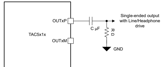
图 6-22. OUT1P 上的单声道单端输出连接 (OUT1x_CFG[2:0] = 3'b010)
