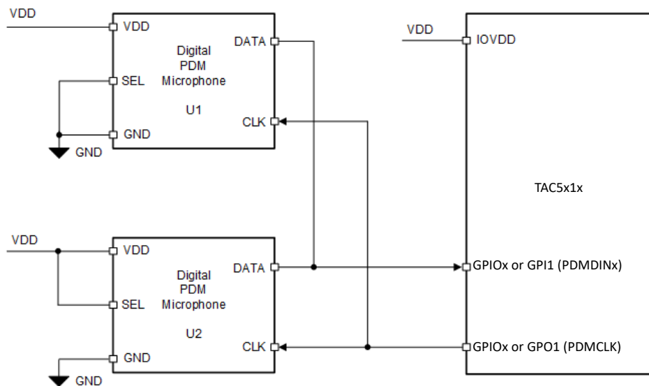
图 6-25. TAC5112-Q1 的数字 PDM 麦克风连接图
