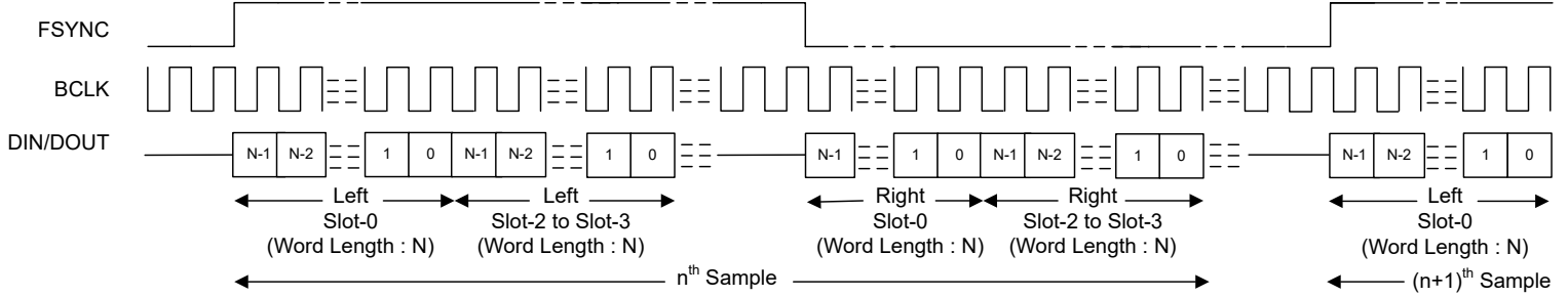
图 6-10. LJ 模式标准协议时序 (TX_OFFSET = 0)
