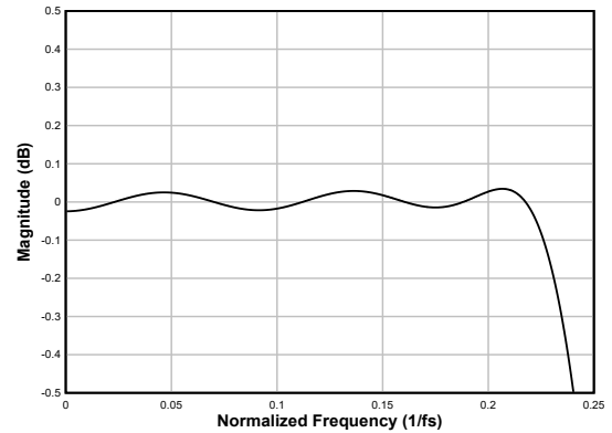
图 6-43. 线性相位抽取滤波器通带纹波
