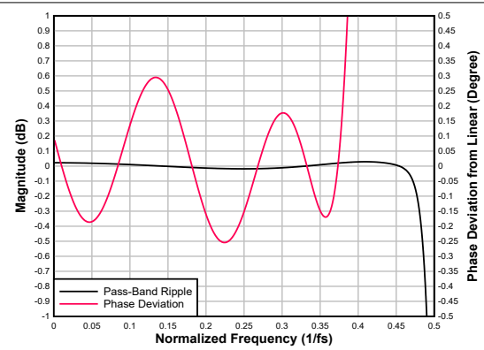
图 6-55. 低延迟抽取滤波器通带纹波和相位偏差
