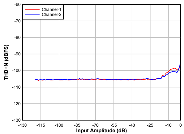
图 6-20. DAC THD+N 级别与输入间的关系
