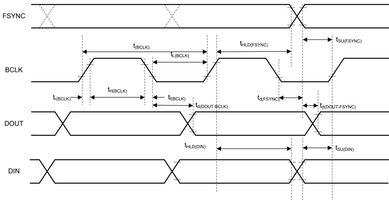
图 6-3. TDM (其中 BCLK_POL = 1)、I²S 和 LJ 接口时序图
