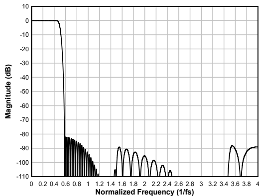
图 7-79. 线性相位内插滤波器幅度响应
