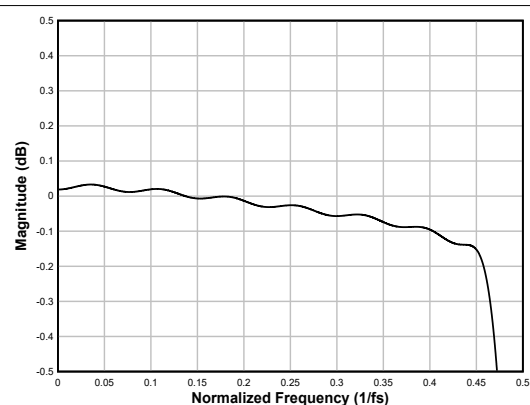
图 7-72. 线性相位内插滤波器通带纹波
