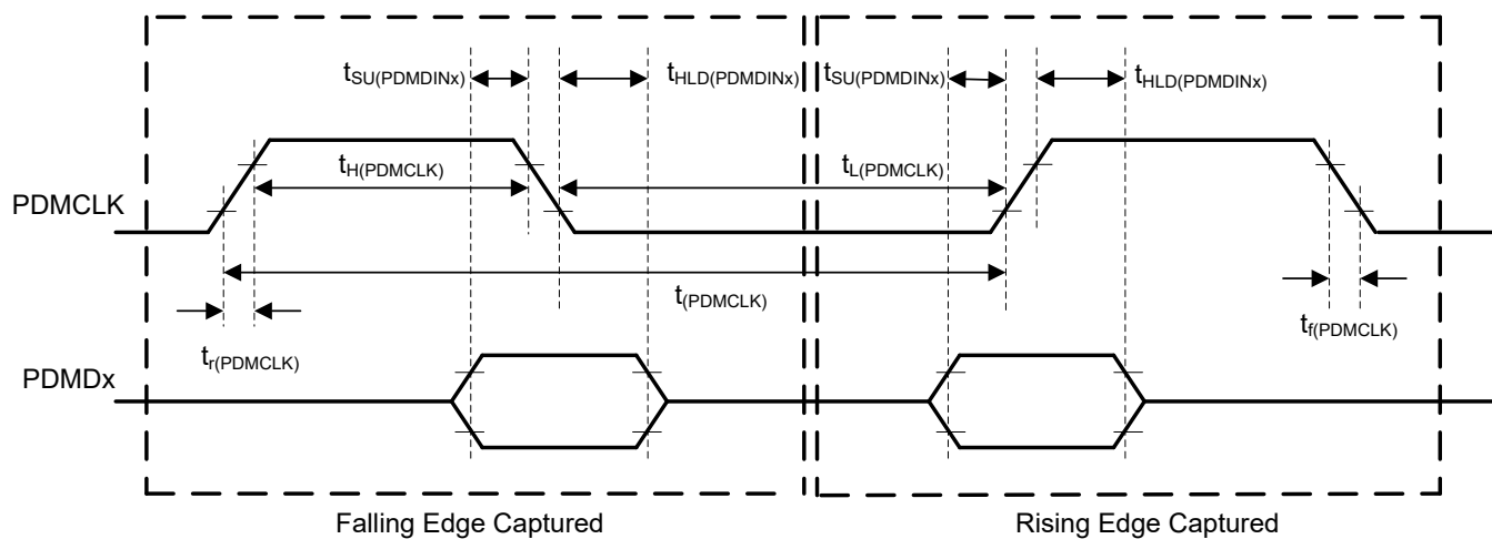
图 6-4. PDM 数字麦克风接口时序图
