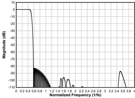
图 7-40. 线性相位抽取滤波器幅度响应
