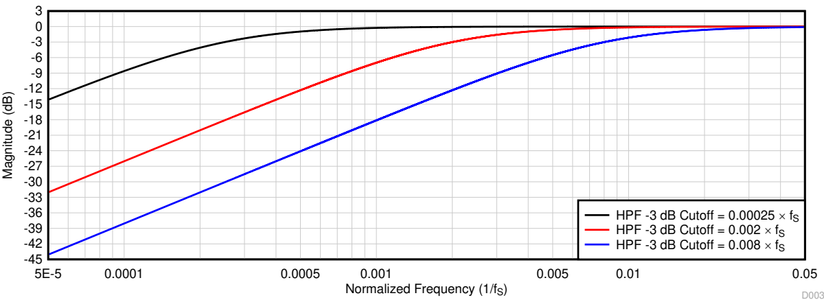
图 7-70. HPF 滤波器频率响应图
