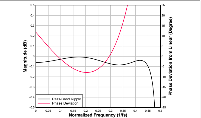
图 7-100. 超低延迟内插滤波器通带纹波和相位偏差
