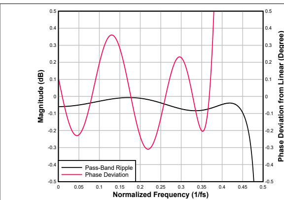
图 7-94. 低延迟内插滤波器通带纹波和相位偏差
