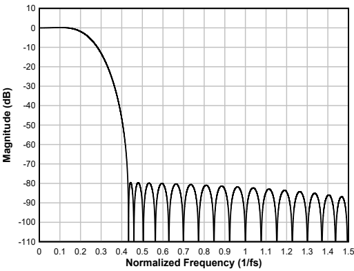
图 7-87. 线性相位内插滤波器幅度响应
