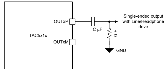
图 7-22. OUT1P 上的单声道单端输出连接 (OUT1x_CFG[2:0] = 3'b010)
