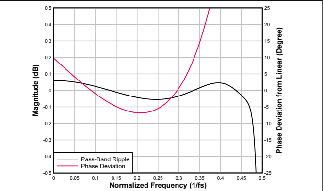
图 7-67. 超低延迟抽取滤波器通带纹波和相位偏差
