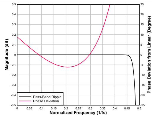
图 7-108. 超低延迟内插滤波器通带纹波和相位偏差
