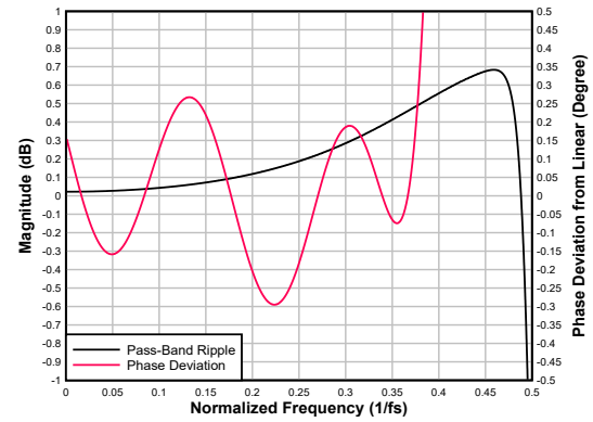
图 7-49. 低延迟抽取滤波器通带纹波和相位偏差
