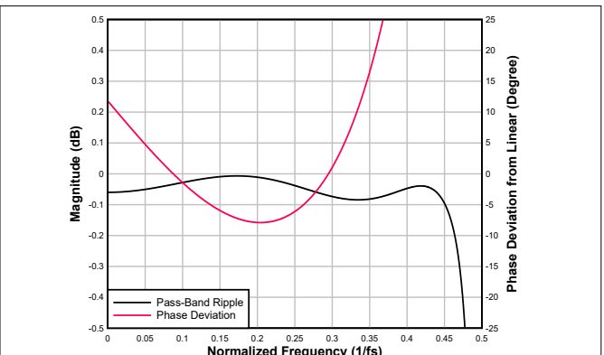
图 7-102. 超低延迟内插滤波器通带纹波和相位偏差
