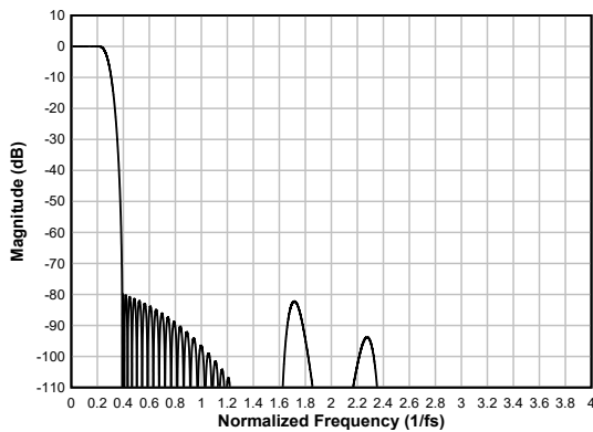
图 7-42. 线性相位抽取滤波器幅度响应
