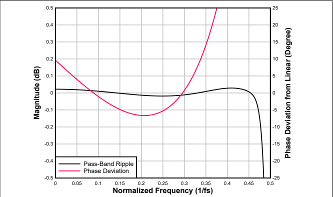
图 7-65. 超低延迟抽取滤波器通带纹波和相位偏差
