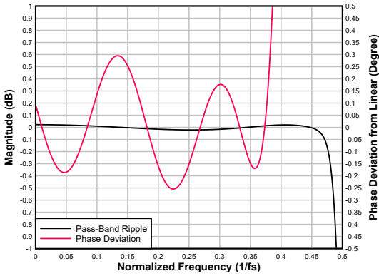
图 7-53. 低延迟抽取滤波器通带纹波和相位偏差
