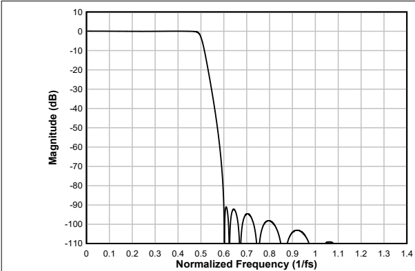
图 7-66. 超低延迟抽取滤波器幅度响应
