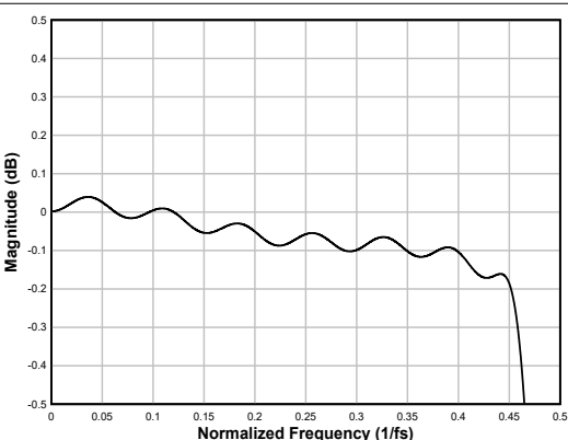
图 7-82. 线性相位内插滤波器通带纹波
