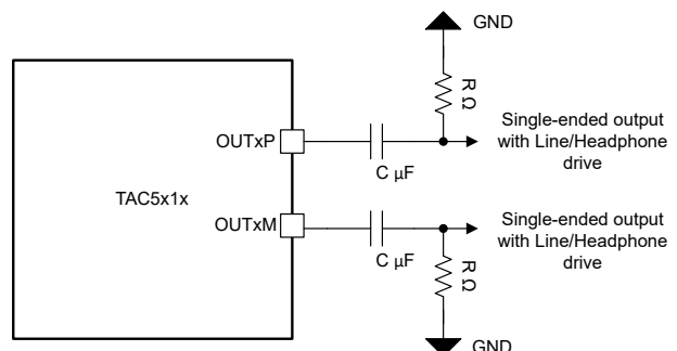
图 7-24. 立体声单端输出连接 (OUT1x_CFG[2:0] = 3'b001)
