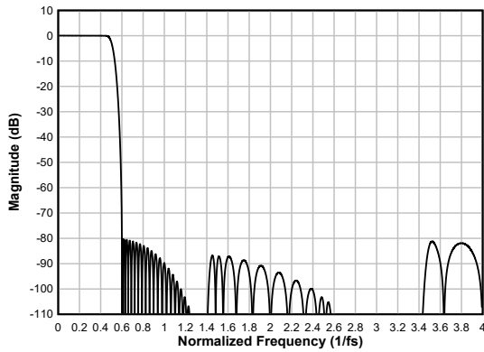
图 7-32. 线性相位抽取滤波器幅度响应
