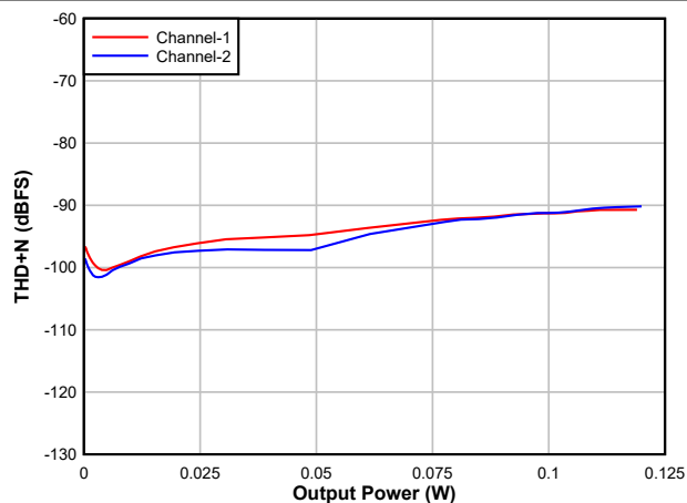
图 6-22. DAC THD+N 级别与输出功率间的关系
