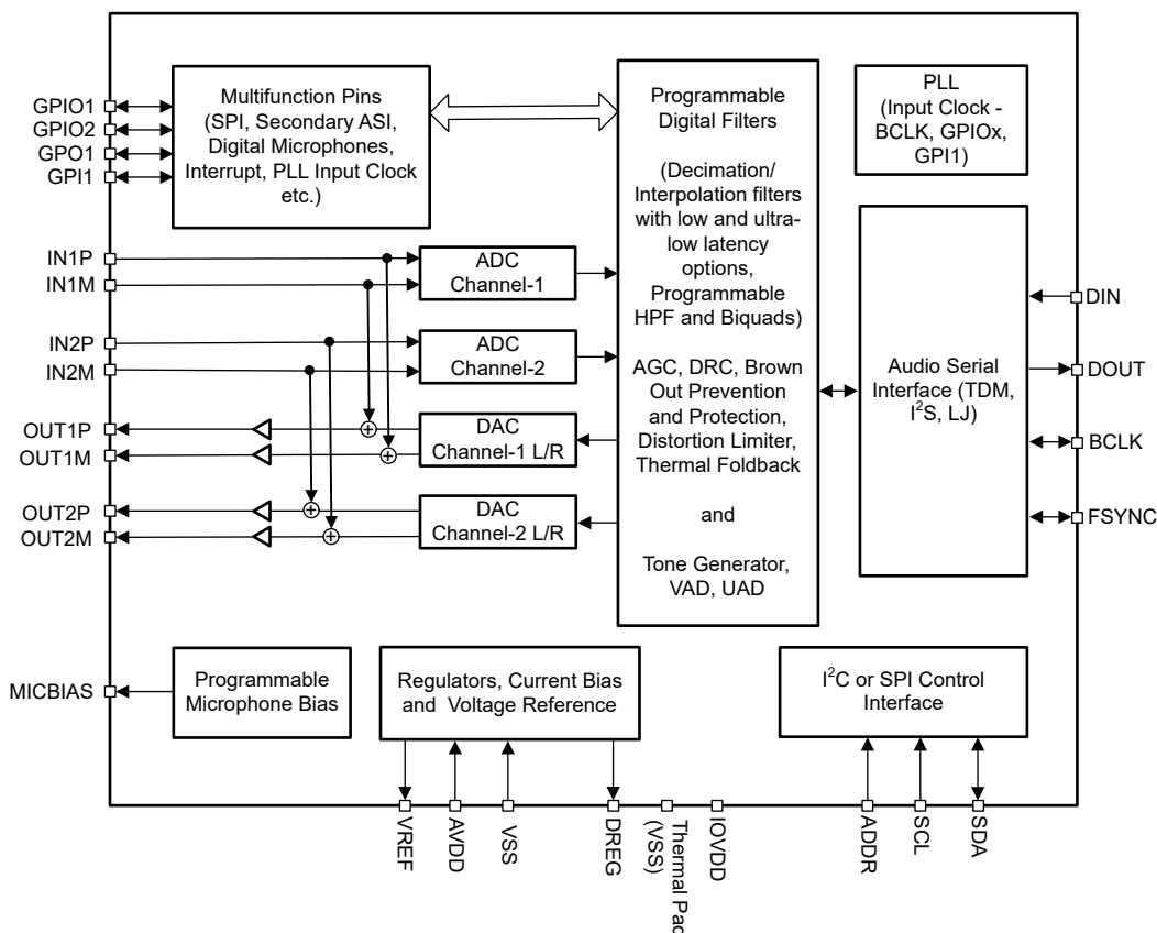
图 7-1. 功能方框图
