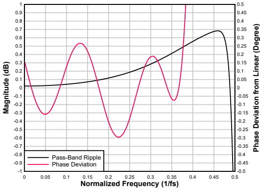
图 7-51. 低延迟抽取滤波器通带纹波和相位偏差
