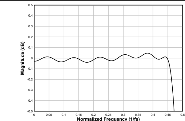
图 7-37. 线性相位抽取滤波器通带纹波
