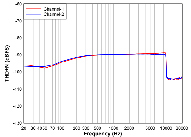
图 6-28. DAC THD+N 级别与频率间的关系
