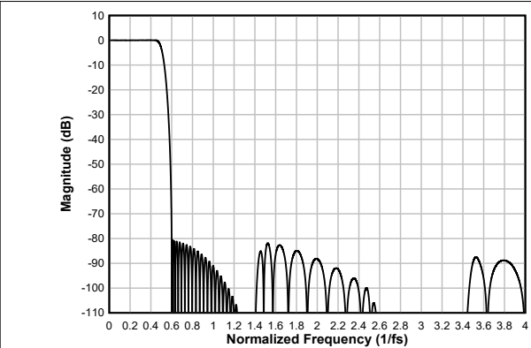
图 7-36. 线性相位抽取滤波器幅度响应
