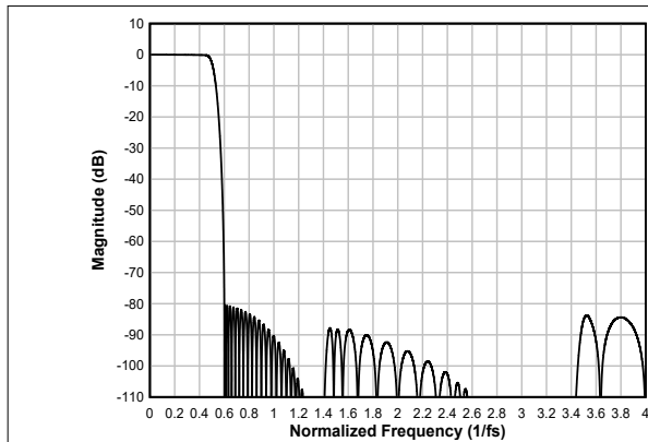
图 7-71. 线性相位内插滤波器幅度响应
