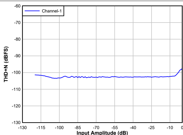
图 5-6. ADC THD+N 级别与输入间的关系
