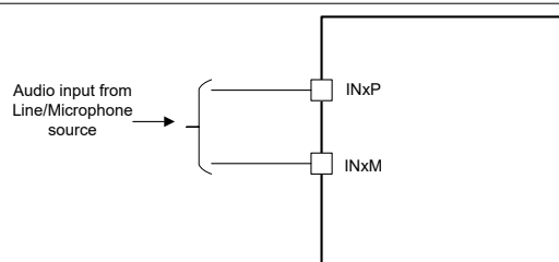
图 6-16. 差分直流耦合输入连接 (ADC_CHx_INSRC 设置为 2'b00、ADC_CHx_CM_TOL 设置为 2'b01 或 2'10)
