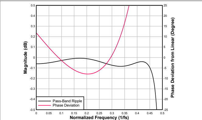
图 6-102. 超低延迟内插滤波器通带纹波和相位偏差
