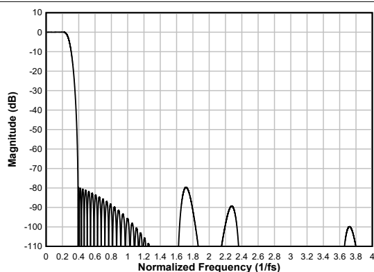
图 6-44. 线性相位抽取滤波器幅度响应
