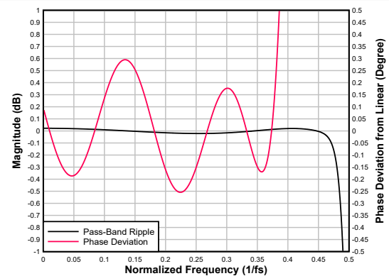
图 6-53. 低延迟抽取滤波器通带纹波和相位偏差
