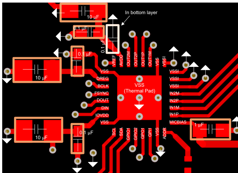
图 8-7. 示例布局
