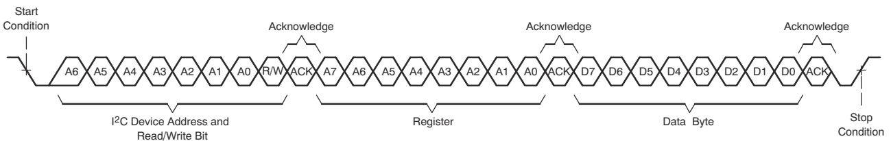
图 6-110. I²C 单字节写入传输
