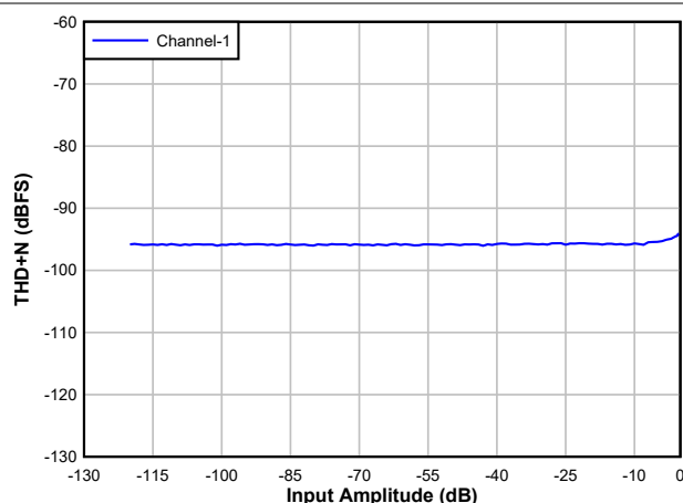
图 5-5. ADC THD+N 级别与输入间的关系
