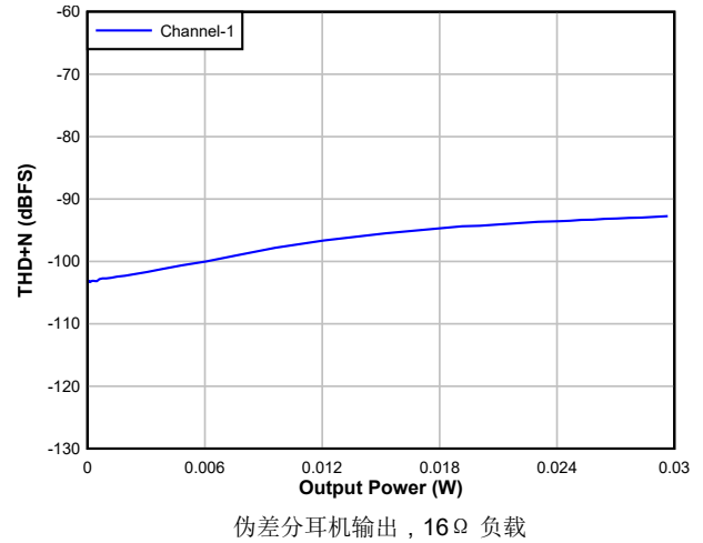
图 5-24. DAC THD+N 级别与输出功率间的关系
