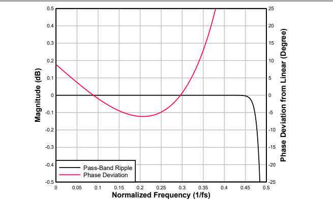
图 6-108. 超低延迟内插滤波器通带纹波和相位偏差
