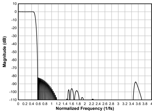
图 6-38. 线性相位抽取滤波器幅度响应
