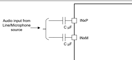
图 6-15. 差分交流耦合输入连接 (ADC_CHx_INSRC 设置为 2'b00、ADC_CHx_CM_TOL 设置为 2'b00 或 2'b01 或 2'10)
