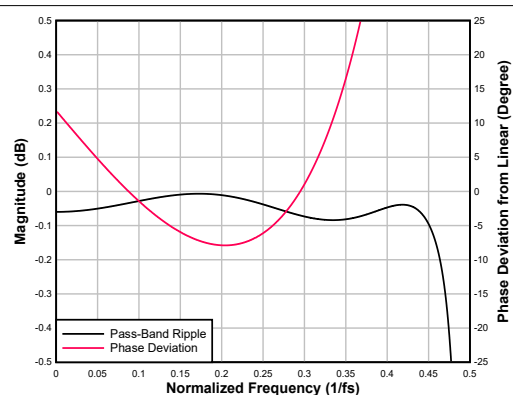
图 6-104. 超低延迟内插滤波器通带纹波和相位偏差
