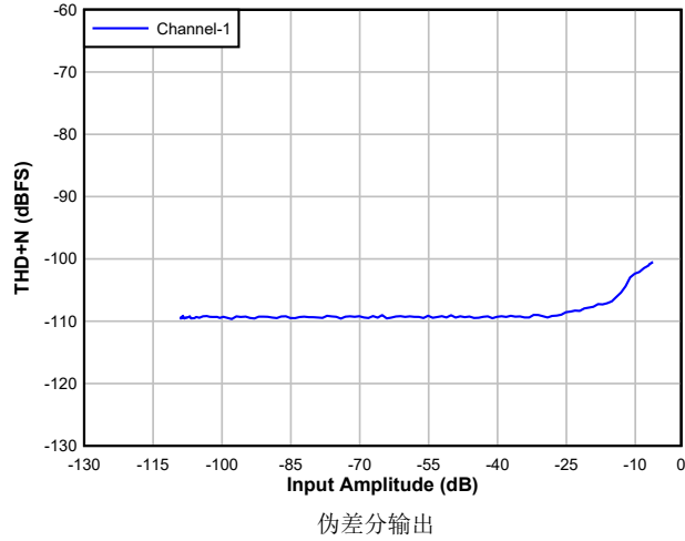
图 5-21. DAC THD+N 级别与输入间的关系
