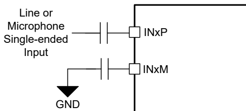
图 6-17. 单端交流耦合输入连接 (ADC_CHx_INSRC 设置为 2'b01、ADC_CHx_CM_TOL 设置为 2'b00 或 2'b01 或 2'10)
