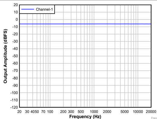
图 5-34. DAC 频率响应
