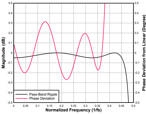
图 6-96. 低延迟内插滤波器通带纹波和相位偏差
