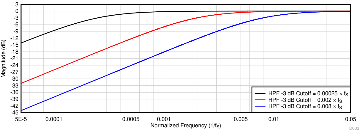
图 6-28. HPF 滤波器频率响应图
