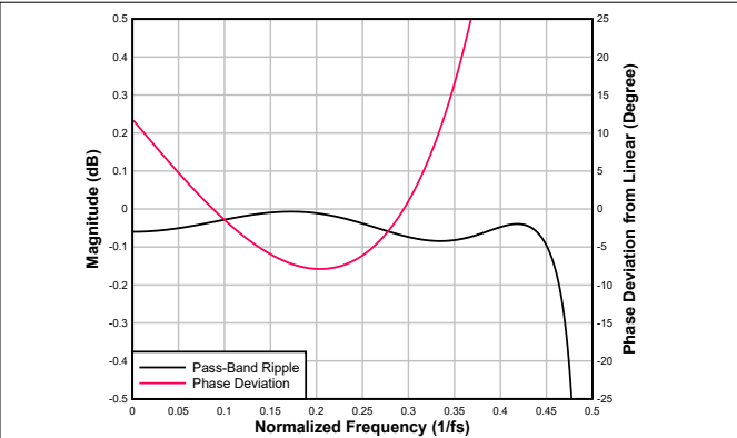
图 6-100. 超低延迟内插滤波器通带纹波和相位偏差
