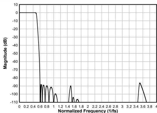
图 6-52. 低延迟抽取滤波器幅度响应
