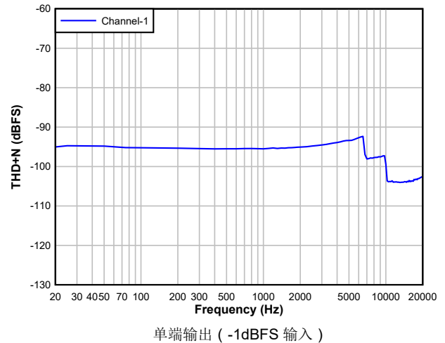
图 5-26. DAC THD+N 级别与频率间的关系
