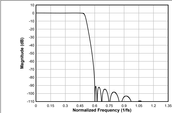
图 6-56. 低延迟抽取滤波器幅度响应
