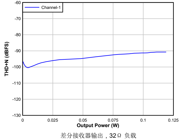
图 5-22. DAC THD+N 级别与输出功率间的关系
