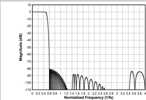
图 6-71. 线性相位内插滤波器幅度响应
