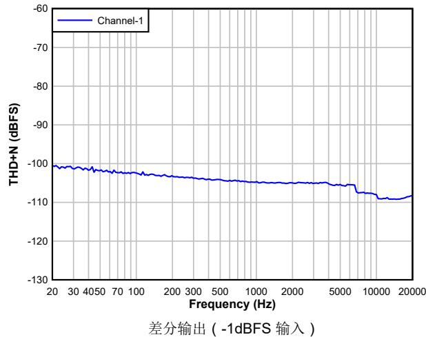
图 5-25. DAC THD+N 级别与频率间的关系
