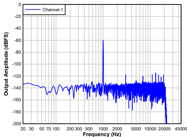
图 5-15. 具有 -60dBFS 输入的 ADC FFT
