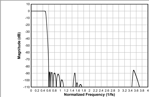
图 6-54. 低延迟抽取滤波器幅度响应
