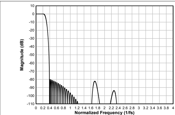
图 6-42. 线性相位抽取滤波器幅度响应
