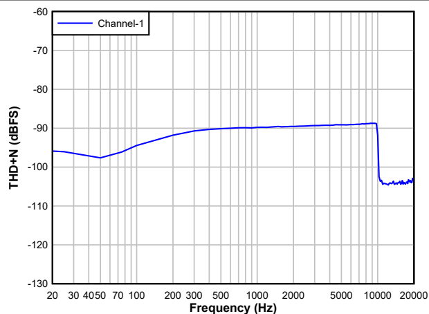
单端耳机输出, 16 \Omega 负载 ( -1dBFS 输入 )
