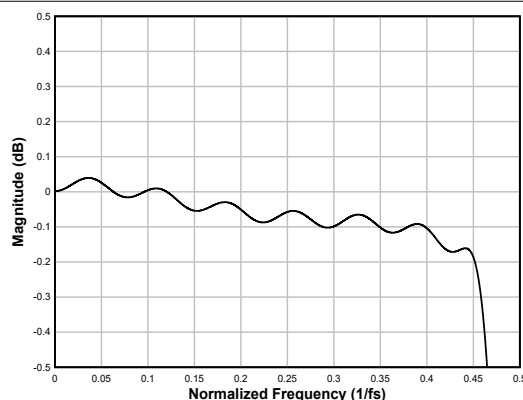
图 6-82. 线性相位内插滤波器通带纹波
