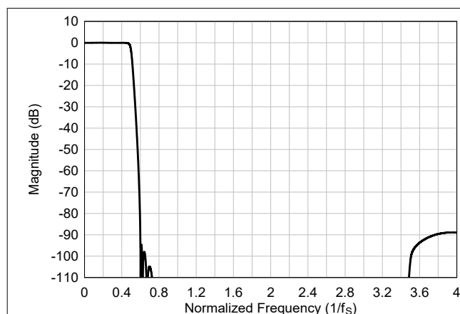
图 6-103. 超低延迟内插滤波器幅度响应
