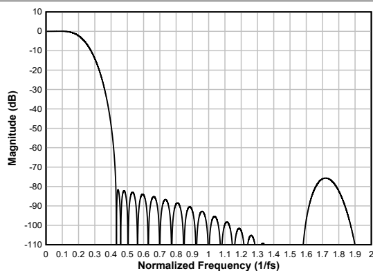
图 6-46. 线性相位抽取滤波器幅度响应
