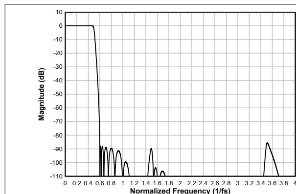
图 6-64. 超低延迟抽取滤波器幅度响应
