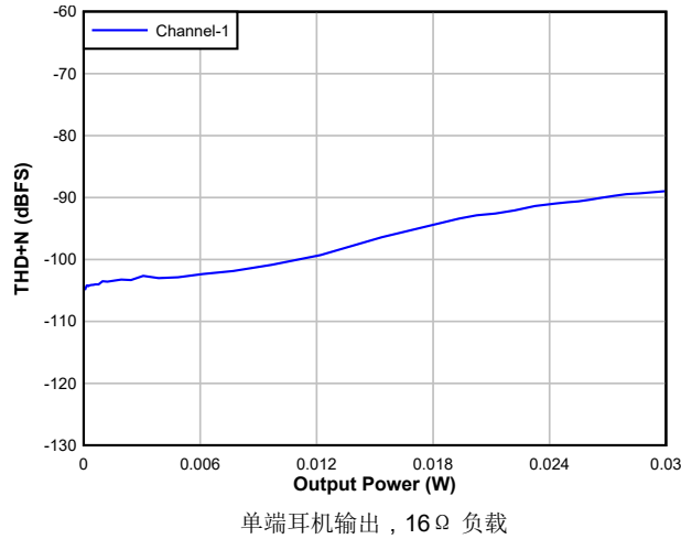
图 5-23. DAC THD+N 级别与输出功率间的关系
