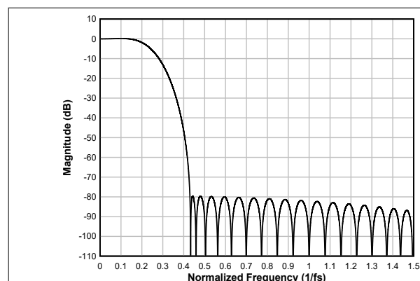
图 6-87. 线性相位内插滤波器幅度响应
