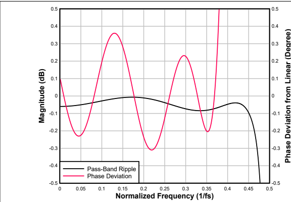
图 6-92. 低延迟内插滤波器通带纹波和相位偏差
