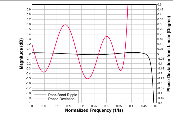
图 6-55. 低延迟抽取滤波器通带纹波和相位偏差
