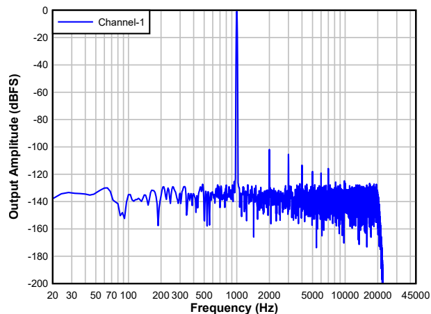
图 5-16. 具有 -1dBFS 输入的 ADC FFT
