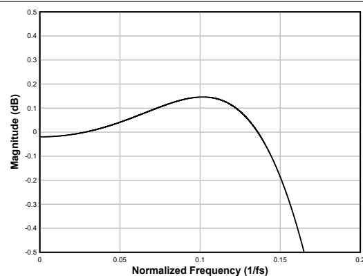
图 6-88. 线性相位内插滤波器通带纹波
