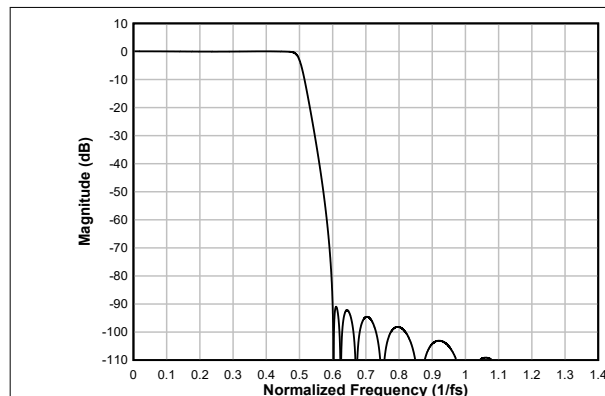
图 6-66. 超低延迟抽取滤波器幅度响应
