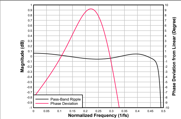
图 6-57. 低延迟抽取滤波器通带纹波和相位偏差
