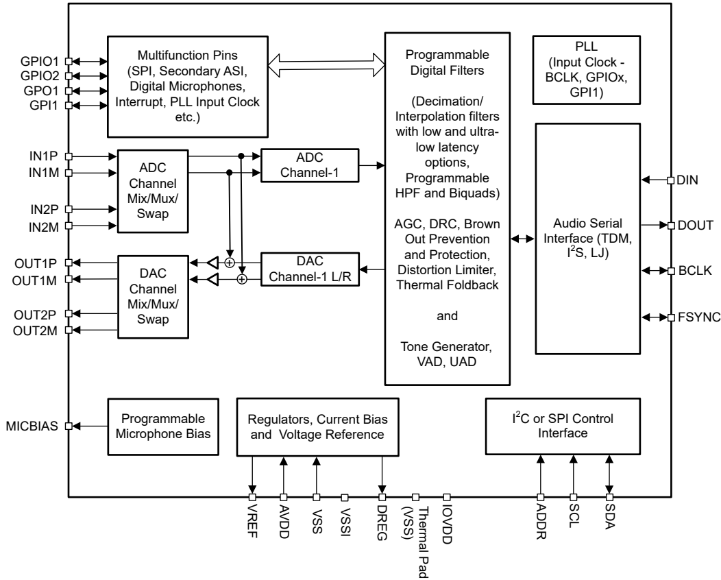
图 6-1. 功能方框图
