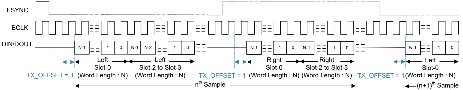
图 7-7. I²S 协议时序 (PASI_TX_OFFSET = 1)
