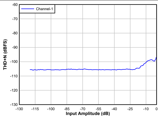
图 6-20. DAC THD+N 级别与输入间的关系
