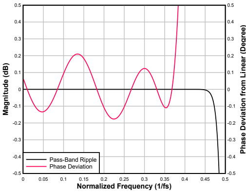
图 7-98. 低延迟内插滤波器通带纹波和相位偏差
