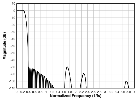
图 7-44. 线性相位抽取滤波器幅度响应
