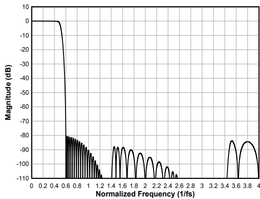
图 7-73. 线性相位内插滤波器幅度响应
