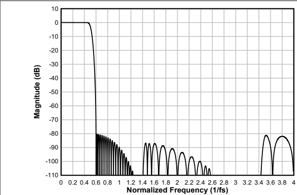
图 7-32. 线性相位抽取滤波器幅度响应
