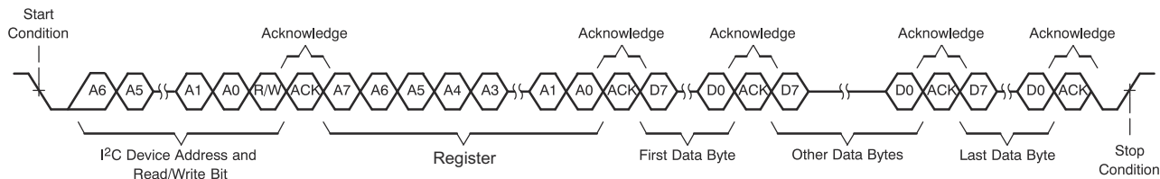
图 7-111. I 2 C 多字节写入传输
