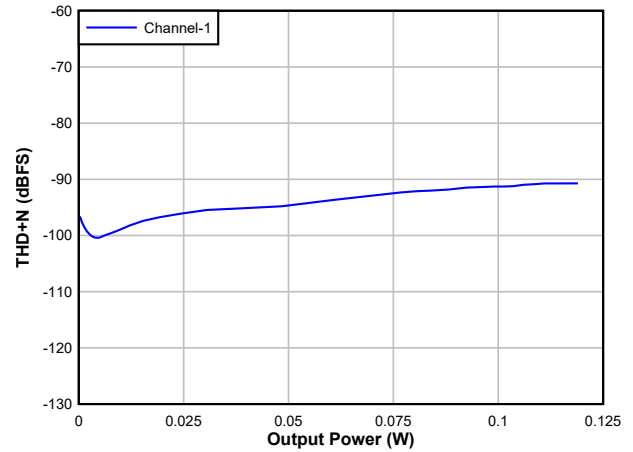
图 6-22. DAC THD+N 级别与输出功率间的关系
