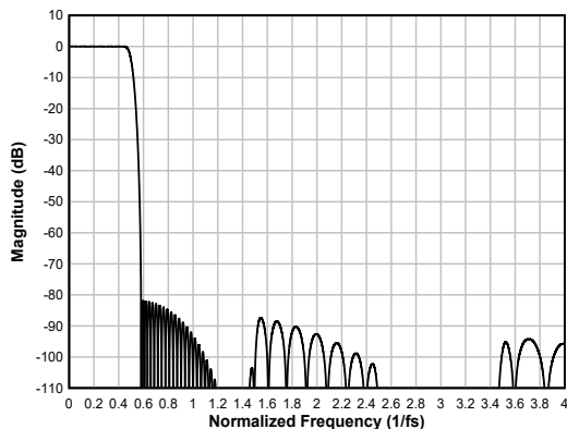
图 7-75. 线性相位内插滤波器幅度响应
