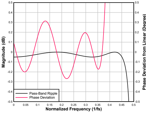
图 7-96. 低延迟内插滤波器通带纹波和相位偏差
