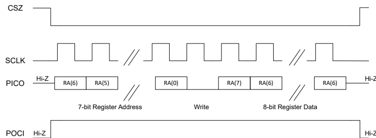
图 7-114. SPI 单字节写入传输
