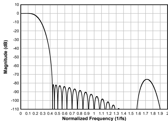
图 7-46. 线性相位抽取滤波器幅度响应
