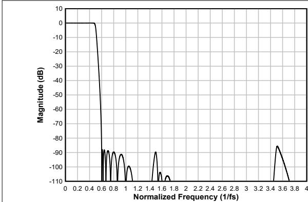
图 7-54. 低延迟抽取滤波器幅度响应
