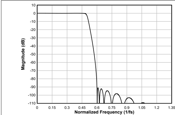
图 7-56. 低延迟抽取滤波器幅度响应
