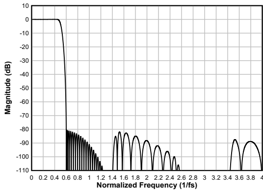
图 7-36. 线性相位抽取滤波器幅度响应
