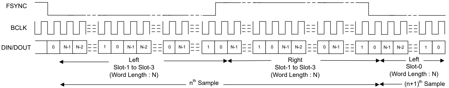
图 7-8. I²S 协议时序 (无空闲 BCLK 周期, PASI_TX_OFFSET = 0)
