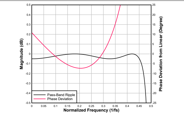
图 7-106. 超低延迟内插滤波器通带纹波和相位偏差
