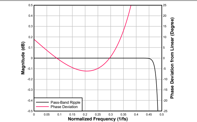
图 7-108. 超低延迟内插滤波器通带纹波和相位偏差
