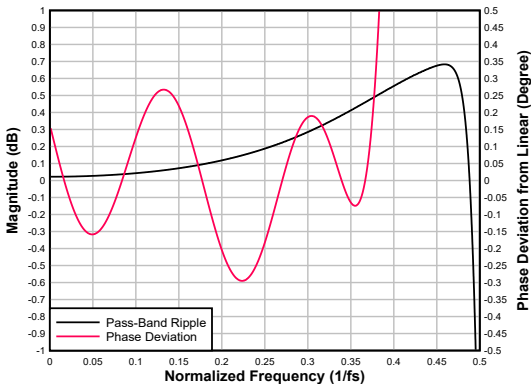
图 7-49. 低延迟抽取滤波器通带纹波和相位偏差
