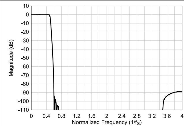
图 7-99. 超低延迟内插滤波器幅度响应
