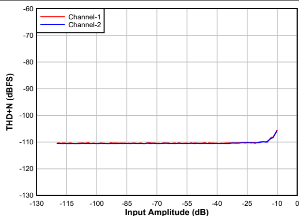
图 8-3. ADC THD+N 级别与输入间的关系
