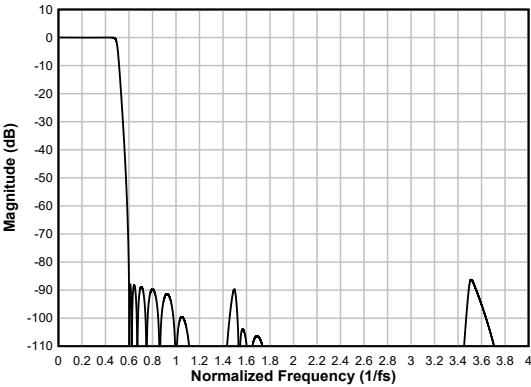
图 6-55. 超低延迟抽取滤波器幅度响应
