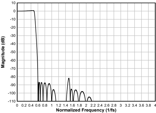
图 6-53. 超低延迟抽取滤波器幅度响应
