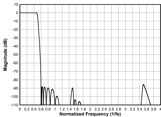
图 6-57. 超低延迟抽取滤波器幅度响应
