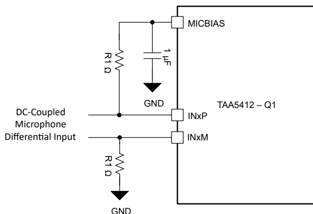
图 6-14. 直流耦合麦克风差分输入连接
