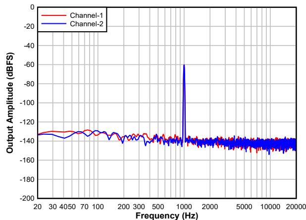
图 8-2. 具有-60dBFS 输入的 ADC FFT
