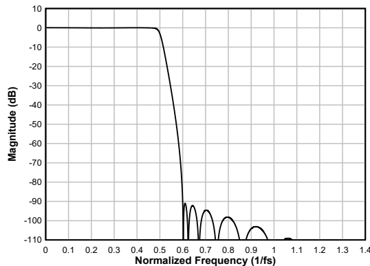
图 6-59. 超低延迟抽取滤波器幅度响应
