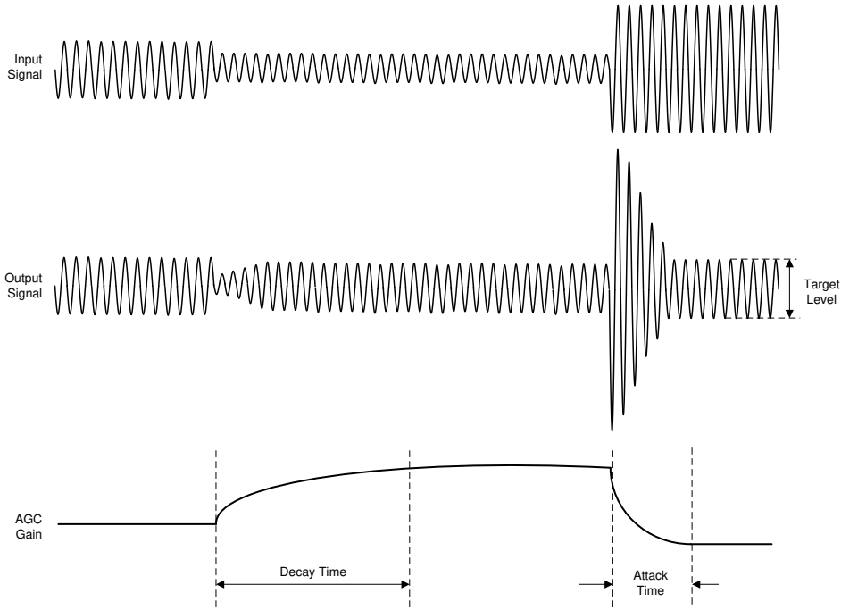
图 6-61. AGC 特性
