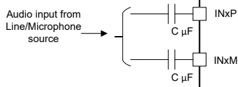
图 6-15. 差分交流耦合输入连接 ( ADC_CHx_INSRC 设置为 2'b00、ADC_CHx_CM_TOL 设置为 2'b00 或 2'b01 或 2'10 )
