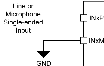
图 6-18. 单端直流耦合输入连接 ( ADC_CHx_INSRC 设置为 2'b01、ADC_CHx_CM_TOL 设置为 2'b01 或 2'10 )
