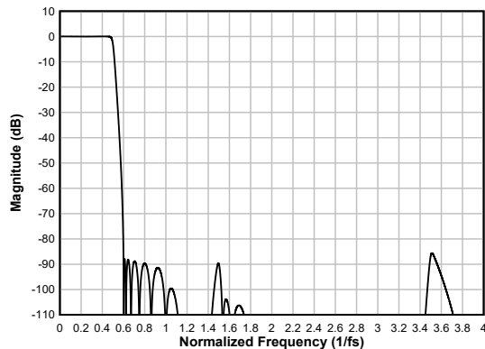
图 6-58. 超低延迟抽取滤波器幅度响应
