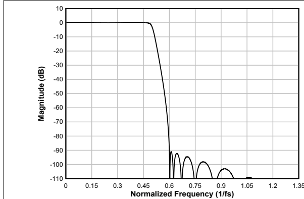
图 6-50. 低延迟抽取滤波器幅度响应
