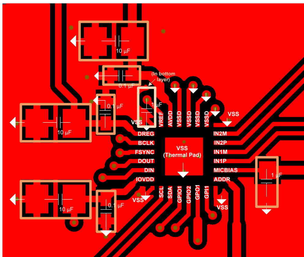
图 8-5. 示例布局
