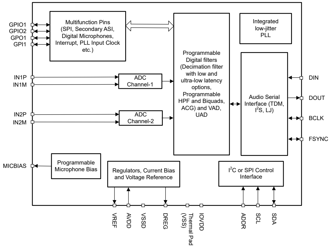
图 6-1. 功能方框图
