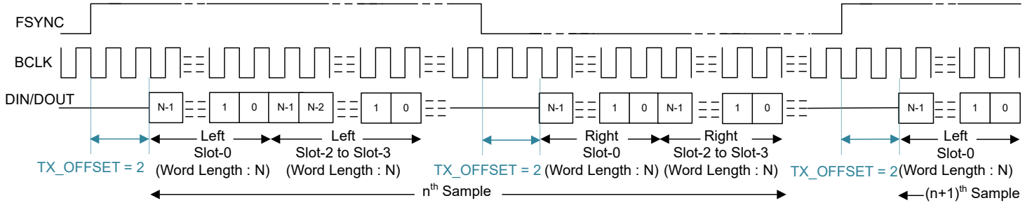
图 6-11. LJ 协议时序 (TX_OFFSET = 2)
