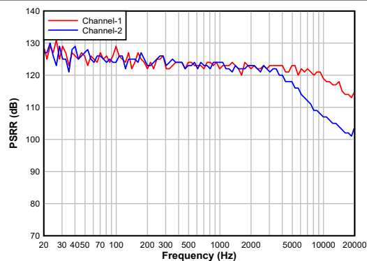
图 5-18. ADC PSRR 与频率间的关系
