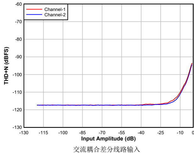
图 8-2. ADC THD + N 级别与输入间的关系
