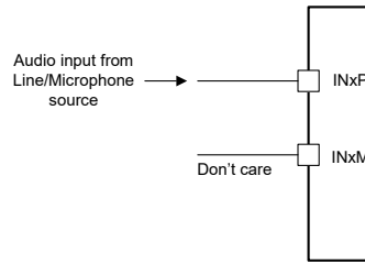
图 6-20. INxP 直流耦合输入连接上的单端多路复用器 ( ADC_CHx_INSRC 设置为 2'b10、ADC_CHx_CM_TOL 设置为 2'b01 或 2'10 )
