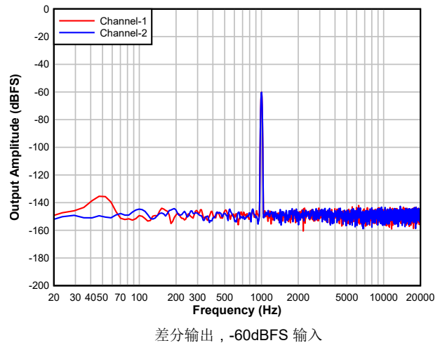
图 8-3. 具有-60dBFS 输入的 ADC FFT
