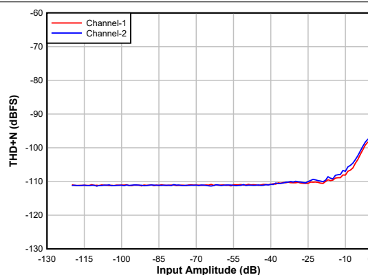
交流耦合差分线路输入， AVDD = 1.8\text{V}
