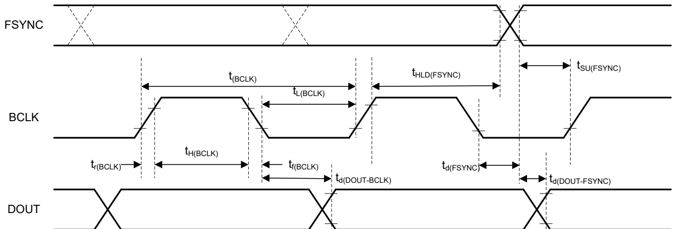
图 5-3. TDM (其中 BCLK_POL = 1)、I²S 和 LJ 接口时序图
