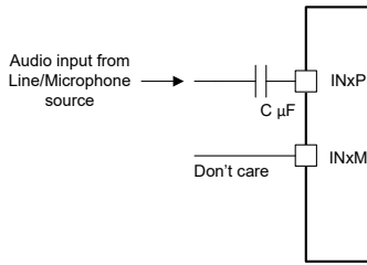
图 6-19. INxP 交流耦合输入连接上的单端多路复用器 ( ADC_CHx_INSRC 设置为 2'b10、ADC_CHx_CM_TOL 设置为 2'b00 或 2'b01 或 2'10 )
