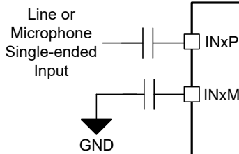
图 6-17. 单端交流耦合输入连接 ( ADC_CHx_INSRC 设置为 2'b01、ADC_CHx_CM_TOL 设置为 2'b00 或 2'b01 或 2'10 )
