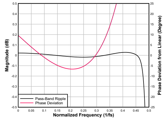
图 6-59. 超低延迟抽取滤波器通带纹波和相位偏差
