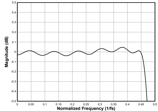
图 6-29. 线性相位抽取滤波器通带纹波
