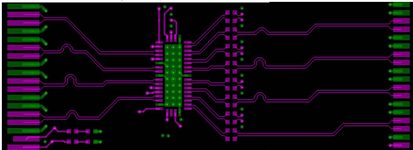
图 7-3. SN75LVPE5421 Layout Example
