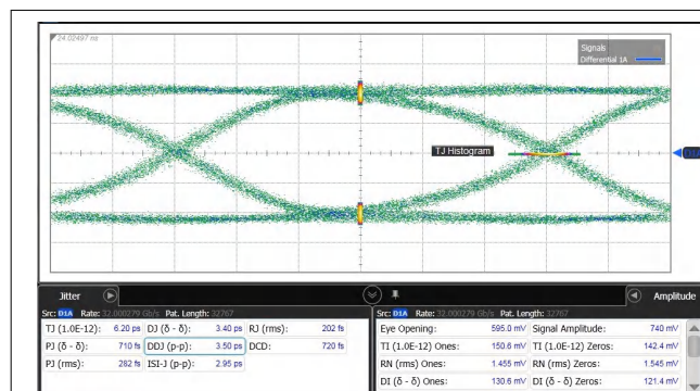
图 5-4. 32 Gbps 800 mV PRBS15 Source (1dB Loss)
