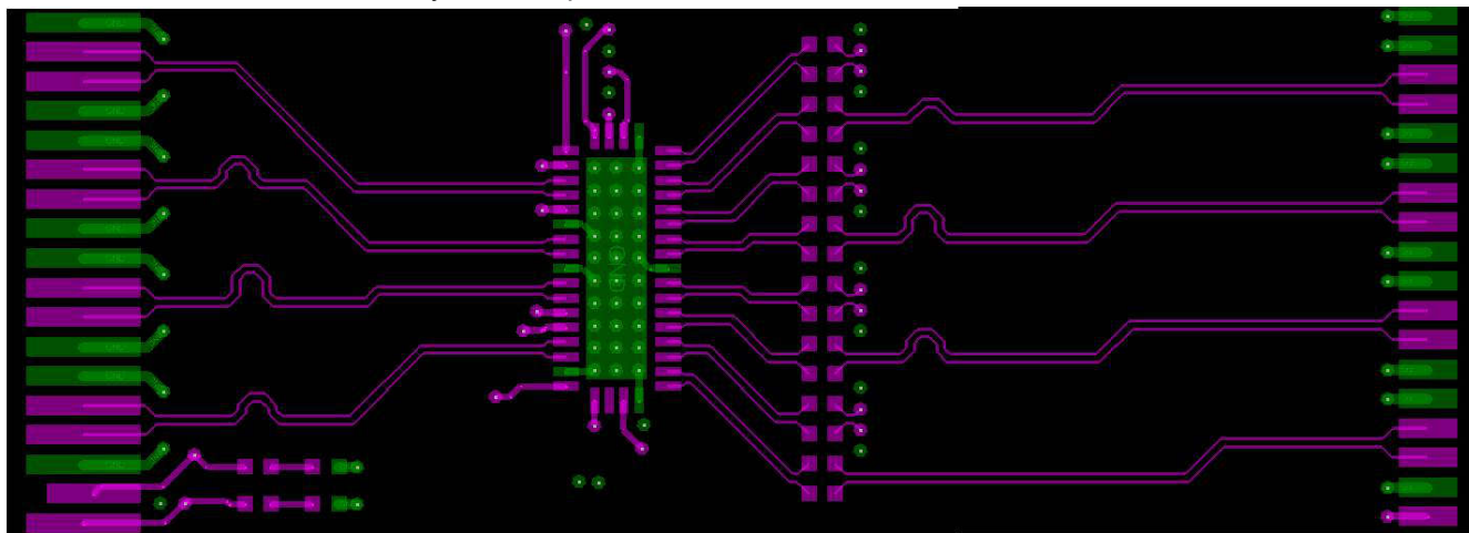
图 7-3. SN75LVPE5412 Layout Example
