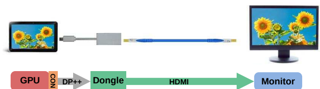
DP159 软件狗应用结构
