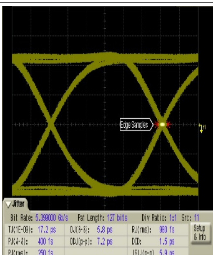
图 30. Eye Diagram (EQ = 10 dB)
