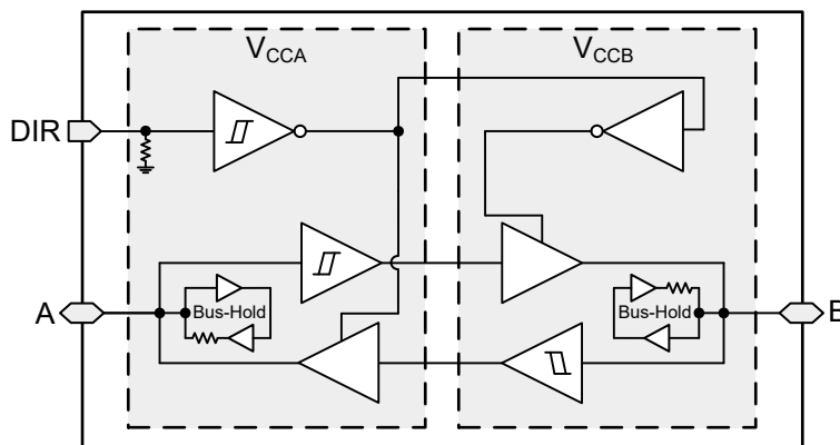
功能方框图
