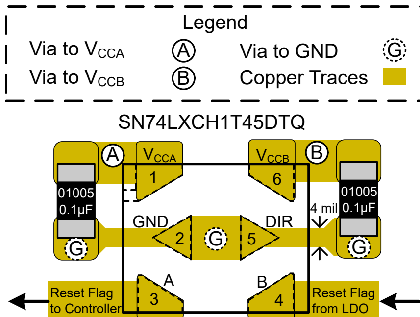
图 11-1. Layout Example
