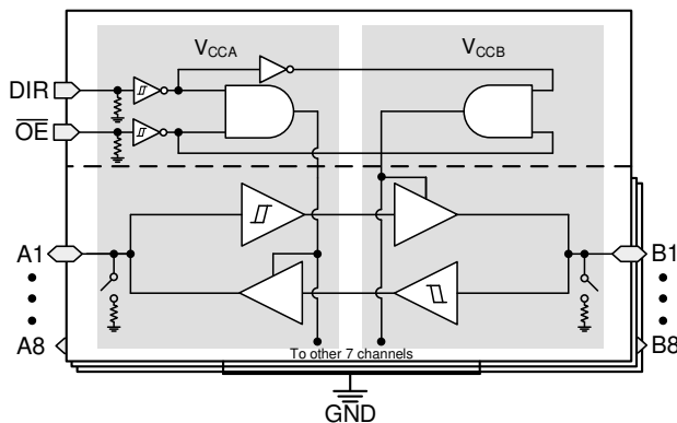
功能方框图
