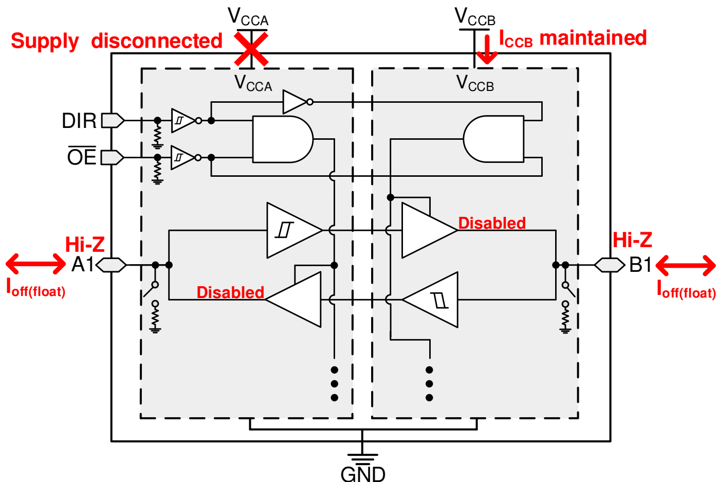
图 8-1. V_{CC} 断开特性
