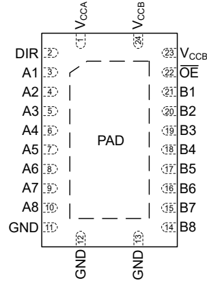
图 5-2. RHL 和 RJW 封装，24 引脚 VQFN 和 UQFN (透明顶视图)
