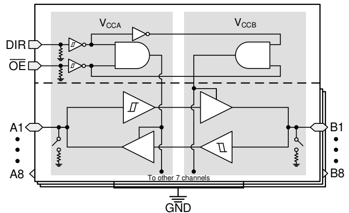
功能方框图
