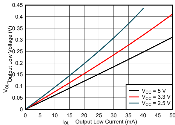
图 6-3. 典型 ( T_A=25^\circ\text{C} ) 输出低电压 ( V_{OL} ) 与灌电流 ( I_{OL} ) 间的关系
