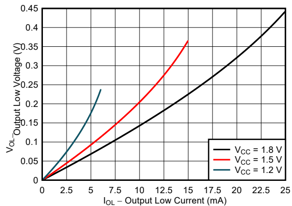
图 6-4. 典型 ( T_A=25^\circ\text{C} ) 输出低电压 ( V_{OL} ) 与灌电流 ( I_{OL} ) 间的关系
