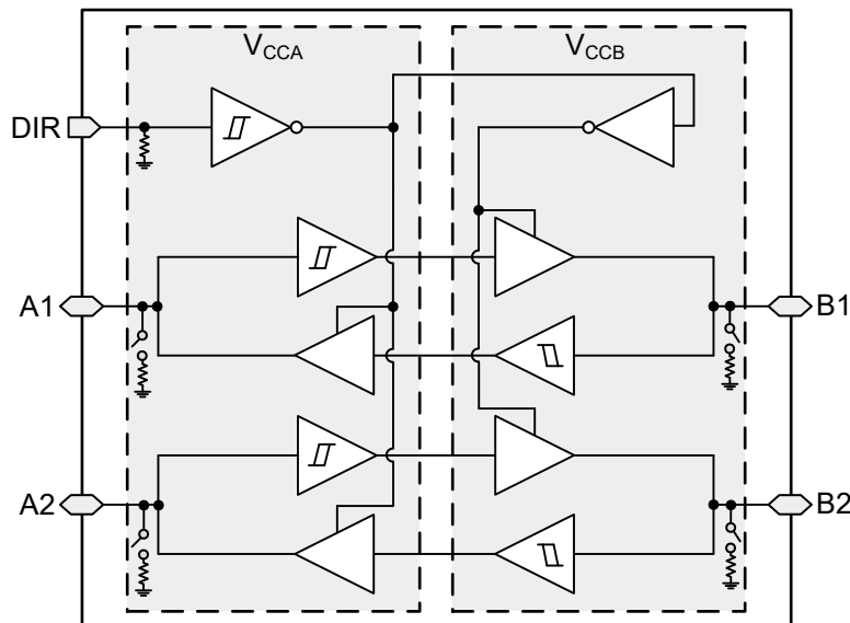
功能方框图
