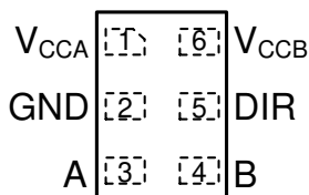
图 5-3. DRY 封装预发布，6 引脚 SON (顶视图)
