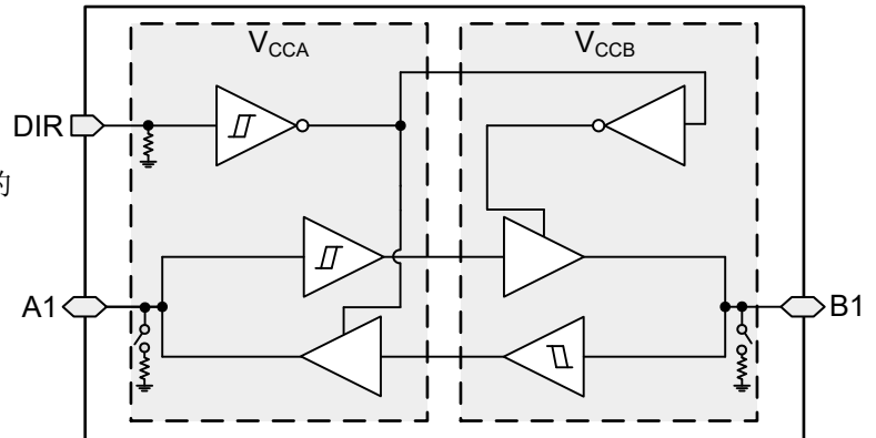
SN74LXC1T45-Q1 框图
