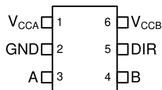
图 5-2. DRL 封装预发布，6 引脚 SOT (顶视图)
