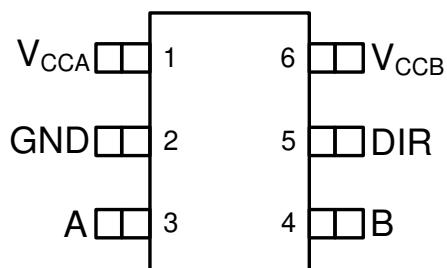
图 5-1. DCK 封装，6 引脚 SC70 (顶视图)
