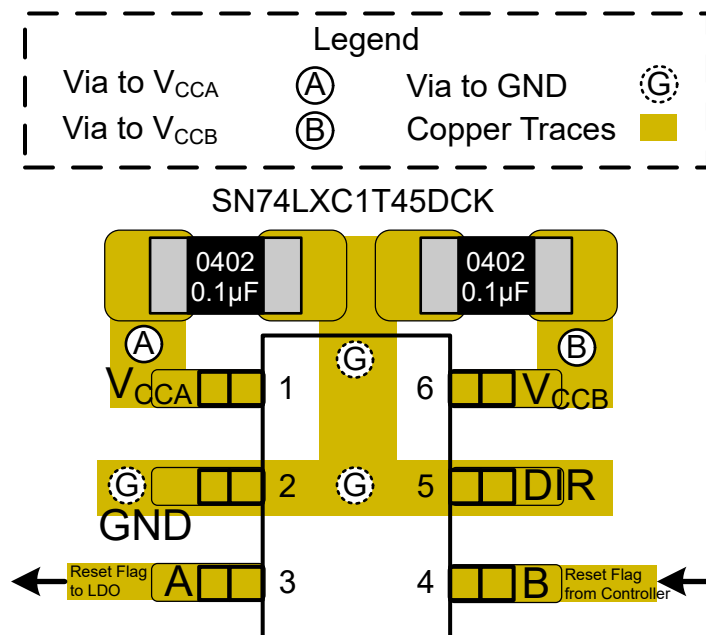
图 11-1. 布局示例 – SN74LXC1T45-Q1
