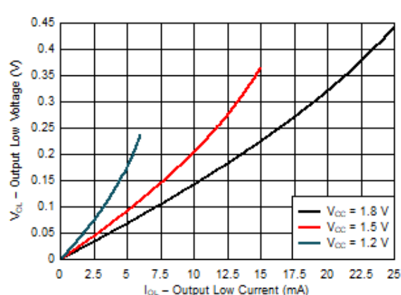
图 6-4. 典型 ( T_A=25^{\circ}\text{C} ) 输出高电压 ( V_{OL} ) 与灌电流 ( I_{OL} ) 间的关系
