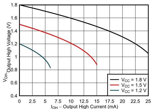
图 6-2. 典型 ( T_A=25^{\circ}\text{C} ) 输出高电压 ( V_{OH} ) 与拉电流 ( I_{OH} ) 间的关系
