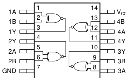
逻辑图
