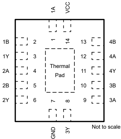
图 4-1. SN74LVC7032A-Q1 BQA Package, 14-Pin WQFN (Top View)
