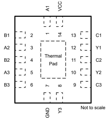
图 4-2. SN74LVC3G57 BQA 封装，14 引脚 WQFN (顶视图)
