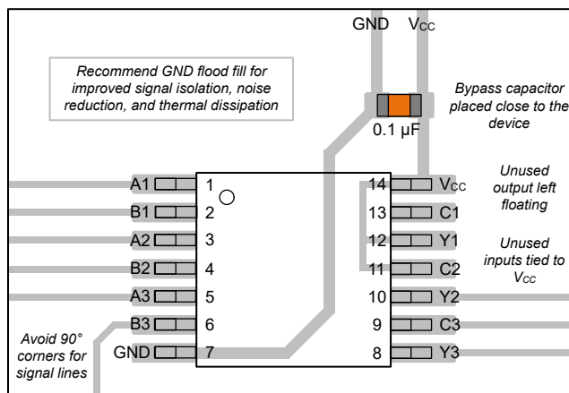
图 8-3. SN74LVC3G57 的示例布局
