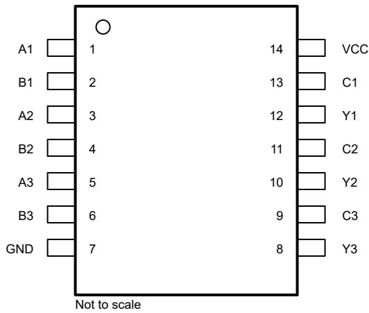
图 4-1. SN74LVC3G57 PW 封装，14 引脚 TSSOP (顶视图)
