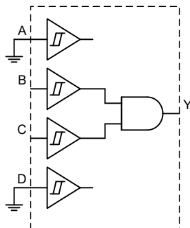
图 7-3. 2 输入与门配置
