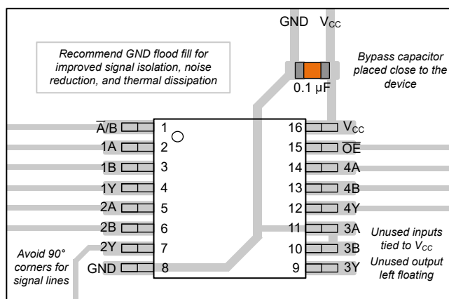
图 8-3. SN74LVC258A 的示例布局
