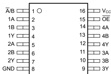
图 4-1. D 或 PW 封装，16 引脚 SOIC 或 TSSOP（顶视图）
