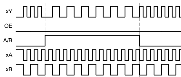
图 8-2. 应用时序图
