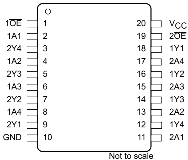
图 4-1. DW、和 PW 封装 20 引脚 SOIC、和 TSSOP 前视图
