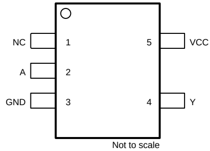
图 4-1. SN74LVC1G16-Q1 DBV 封装，5 引脚 SOT-23 ( 顶视图 )
