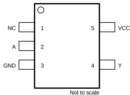
图 4-2. SN74LVC1G16 DCK 封装，5 引脚 SOT-SC70 (顶视图)
