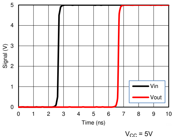
图 8-2. 显示传播延迟的模拟输入至输出电压响应
