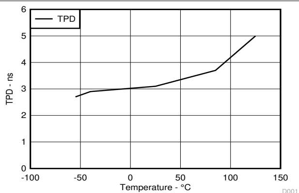
图 5-1. 3.3V V_{CC} 时 TPD 与温度间的关系
