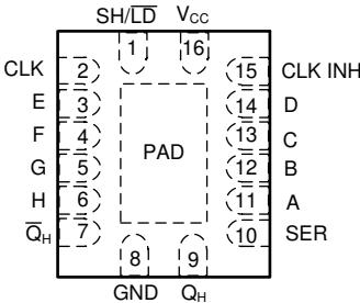
图 4-1. BQB 封装，16 引脚 WQFN（顶视图）
