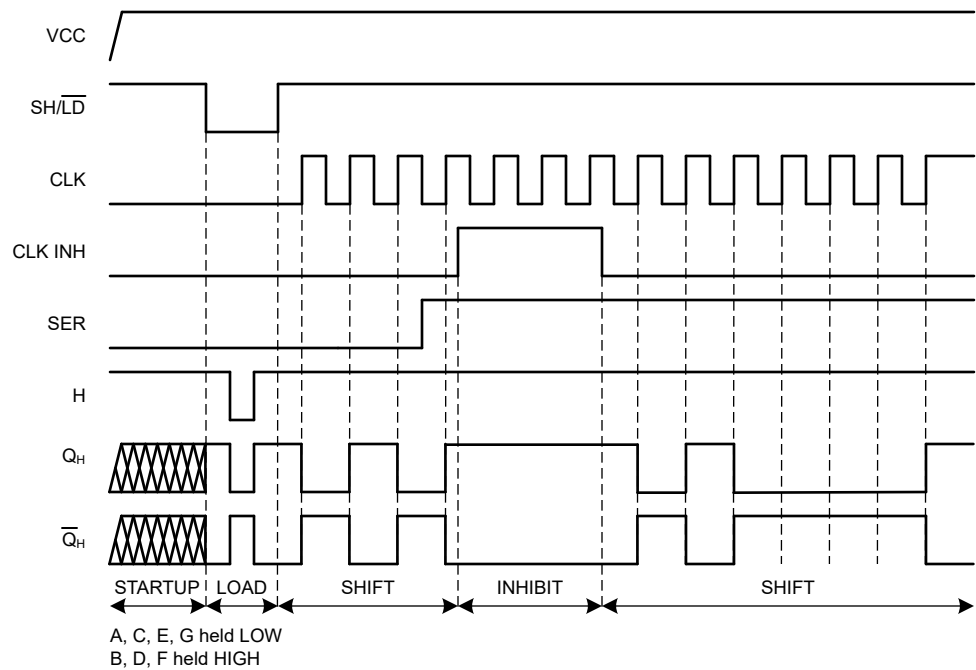
图 5-1. 时序图
