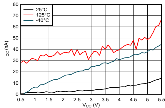
图 5-4. 电源电压两端的电源电流
