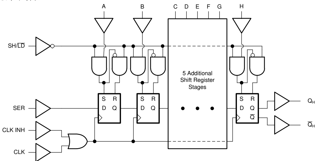
功能图
