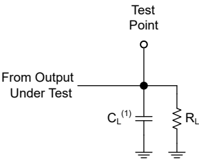
图 6-1. 推挽输出的负载电路
