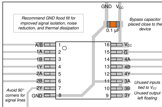
图 8-3. SN74LVC158A 的示例布局
