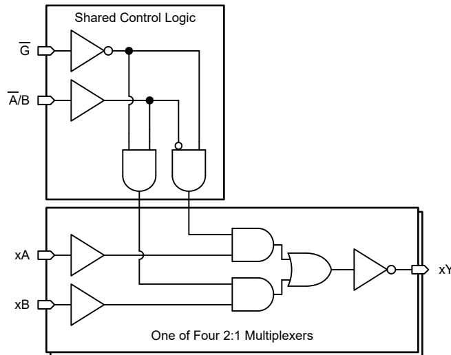
图 7-1. SN74LVC158A 的逻辑图 (正逻辑)
