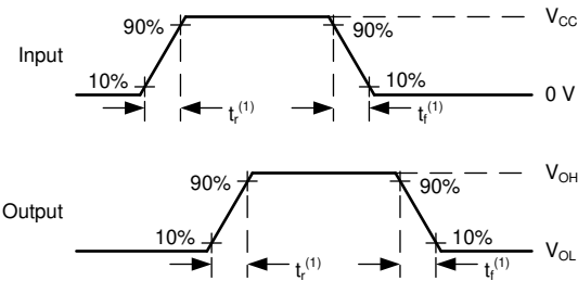
图 6-3. 电压波形，输入和输出转换时间
