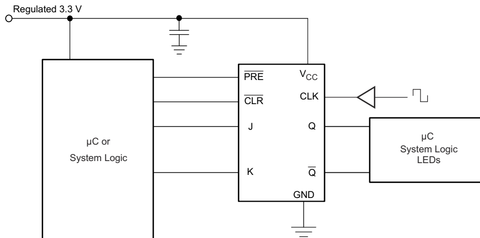
图 8-1. 典型应用原理图
