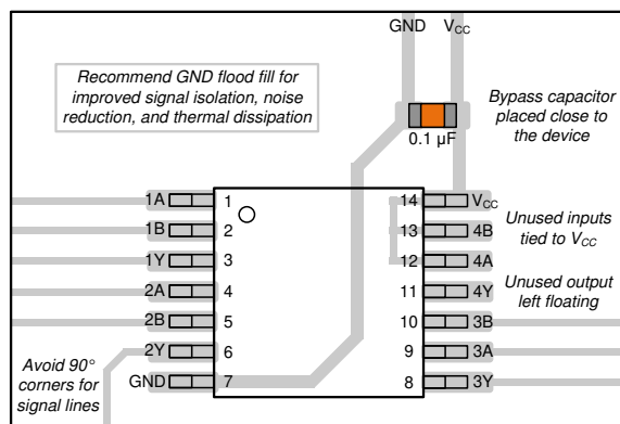
图 7-1. Example Layout for the SN74LVC08A-Q1
