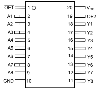
图 4-2. SN74LV8T9541-Q1 PW、DGS 封装 (顶视图)
