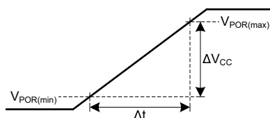
图 7-2. 已知上电状态的电源 ( V_{CC} ) 斜坡特性
