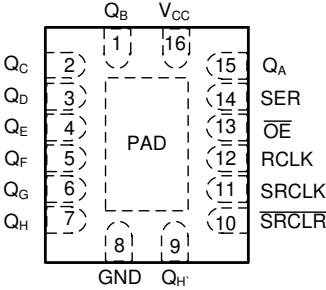
图 4-2. BQB 封装，16 引脚 WQFN ( 透明顶视图 )
