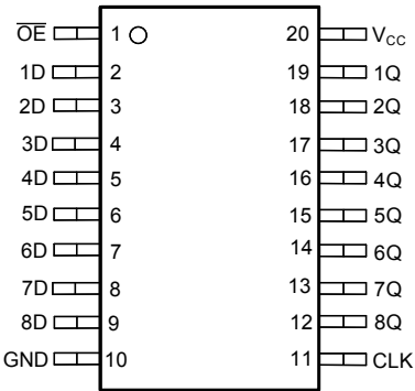
图 4-2. SN74LV8T574-Q1 PW、DGS 封装 (顶视图)
