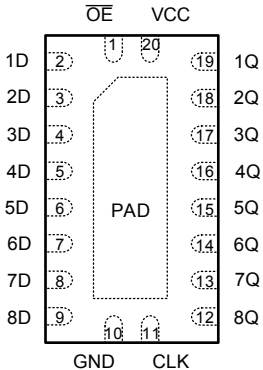
图 4-1. SN74LV8T574-Q1 RKS 封装 (顶视图)
