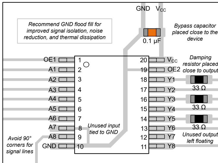
图 10-3. SN74LV8T541-Q1 采用 TSSOP 封装的示例布局
