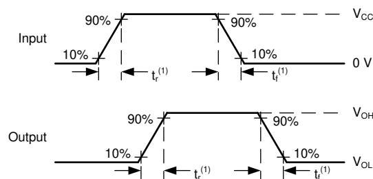
图 6-4. 电压波形，输入和输出转换时间
