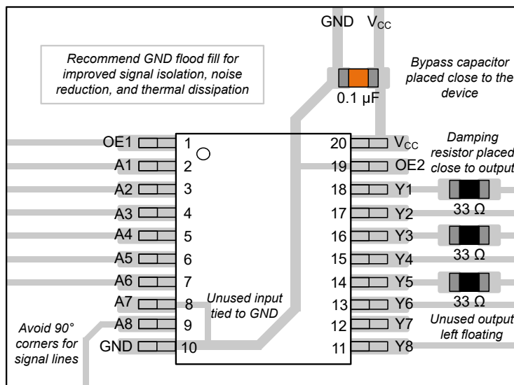
图 10-3. SN74LV8T541 采用 TSSOP 封装的示例布局
