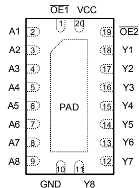
图 4-2. RKS 封装，20 引脚 VQFN (透明顶视图)
