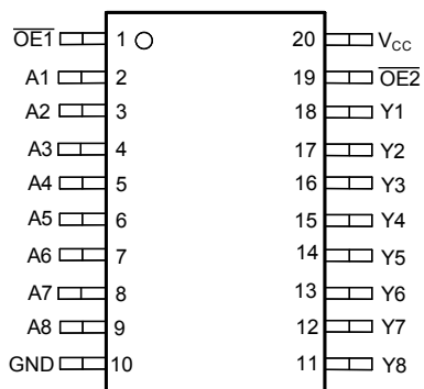
图 4-1. PW 和 DGS 封装，20 引脚 TSSOP (顶视图)
