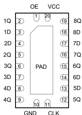
图 4-1. SN74LV8T374-Q1 RKS 封装 (顶视图)
