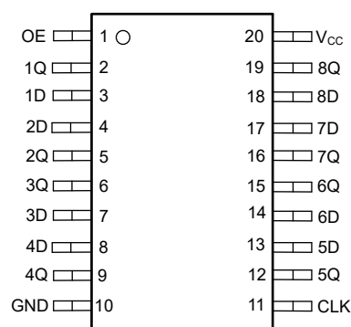
图 4-2. SN74LV8T374-Q1 PW、DGS 封装 (顶视图)
