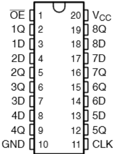
图 7-1. PW 封装 20 引脚 TSSOP ( 顶视图 )
