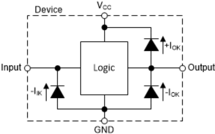
图 8-4. 每个输入和输出的钳位二极管的电气布置
