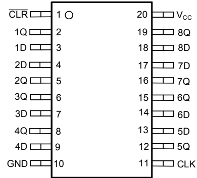
图 4-2. SN74LV8T273-Q1 PW、DGS 封装 (顶视图)
