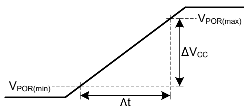
图 7-1. 已知上电状态的电源 (V CC ) 斜坡特性
