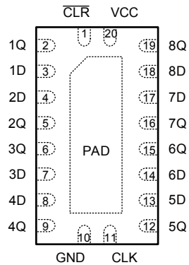
图 4-1. SN74LV8T273 RKS 封装 (顶视图)
