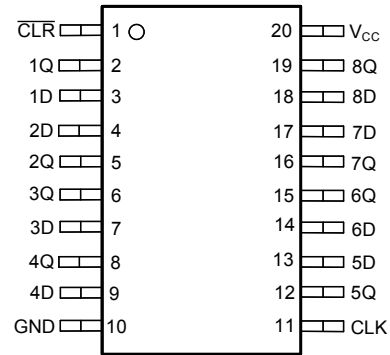
图 4-2. SN74LV8T273 PW、DGS 封装 (顶视图)
