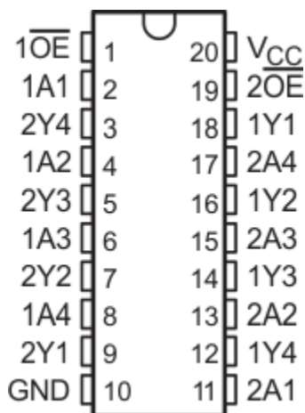
图 4-1. SN74LV240A PW 封装；20 引脚 TSSOP（顶视图）
