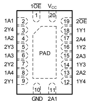
图 4-2. SN74LV8T240 RKS 封装；20 引脚 TSSOP (顶视图)
