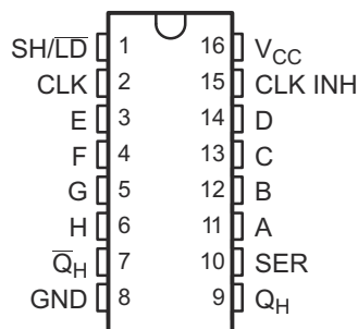
图 4-1. PW 封装， 16 引脚 TSSOP (顶视图)
