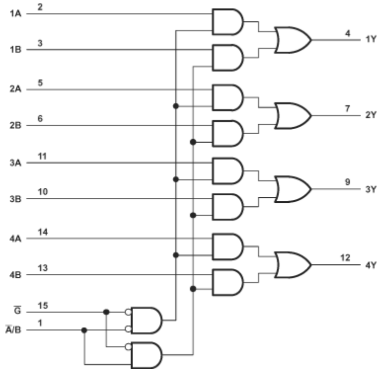
图 7-1. 逻辑图 (正逻辑)
