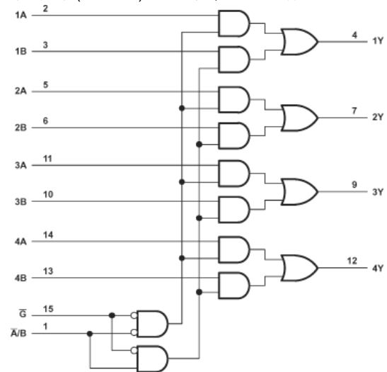
逻辑图 (正逻辑)
