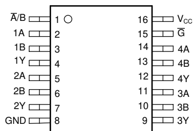
图 4-1. PW 封装 ( 顶视图 )
