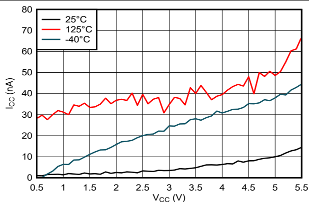
图 7-3. 电源电压两端的电源电流
