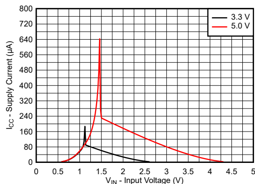
图 7-2. 3.3V 和 5.0V 输入电压电源上的电源电流
