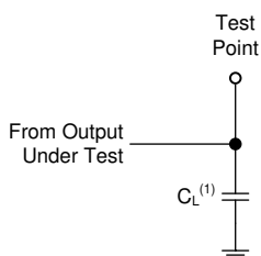
图 8-1. 推挽输出的负载电路
