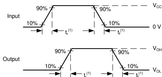
图 8-3. 电压波形，输入和输出转换时间
