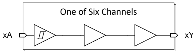
简化逻辑图 (正逻辑)
