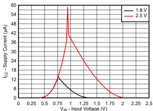
图 7-1. 1.8V 和 2.5V 输入电压电源上的电源电流
