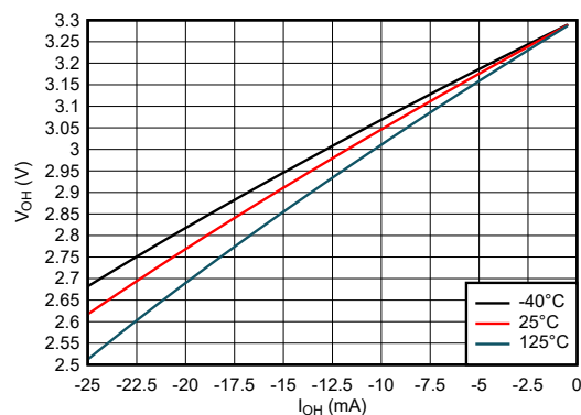
图 7-8. 高电平状态下输出电压与电流间的关系；3.3V 电源
