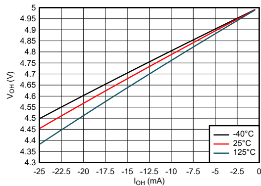
图 7-6. 高电平状态下输出电压与电流间的关系 (5V 电源)
