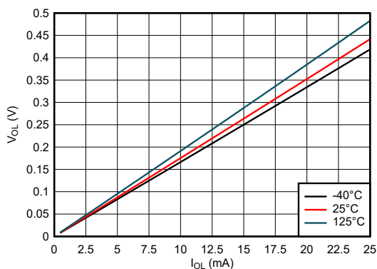
图 7-7. 低电平状态下输出电压与电流间的关系；5V 电源
