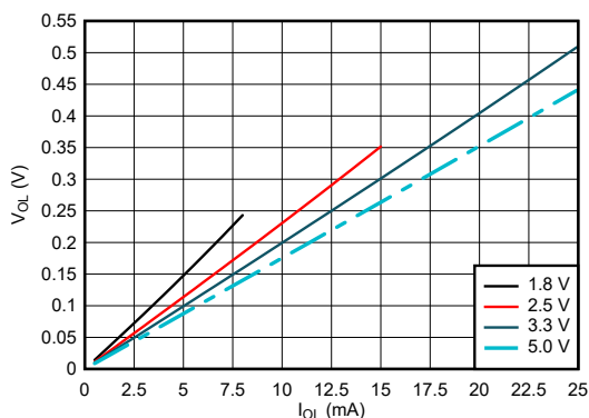
图 7-5. 低电平状态下输出电压与电流间的关系
