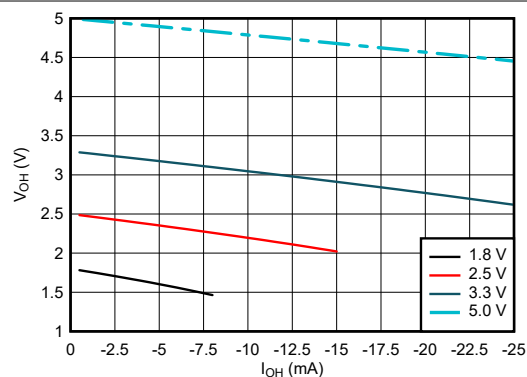
图 7-4. 高电平状态下输出电压与电流间的关系
