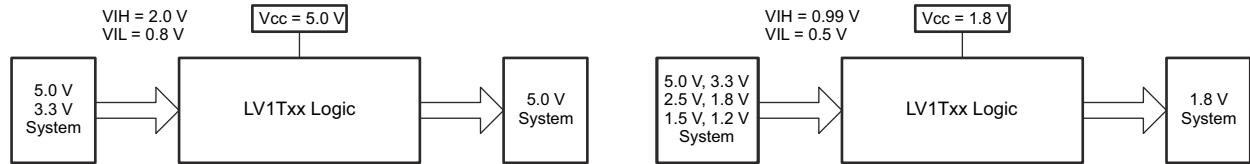
图 9-3. LVxT 升压和降压转换示例
